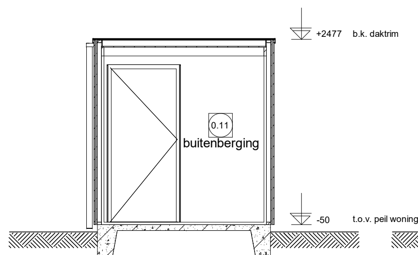
Doorsnede E
