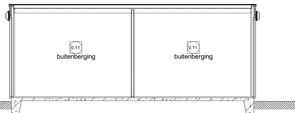
Doorsnede F
