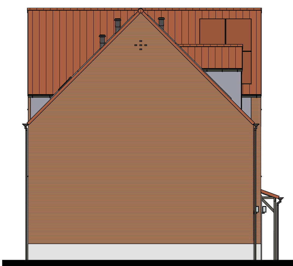
Linkergevel
