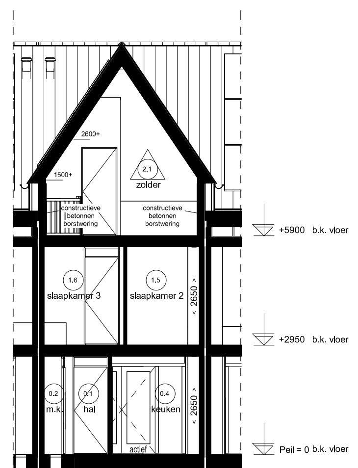
Doorsnede B02.2
