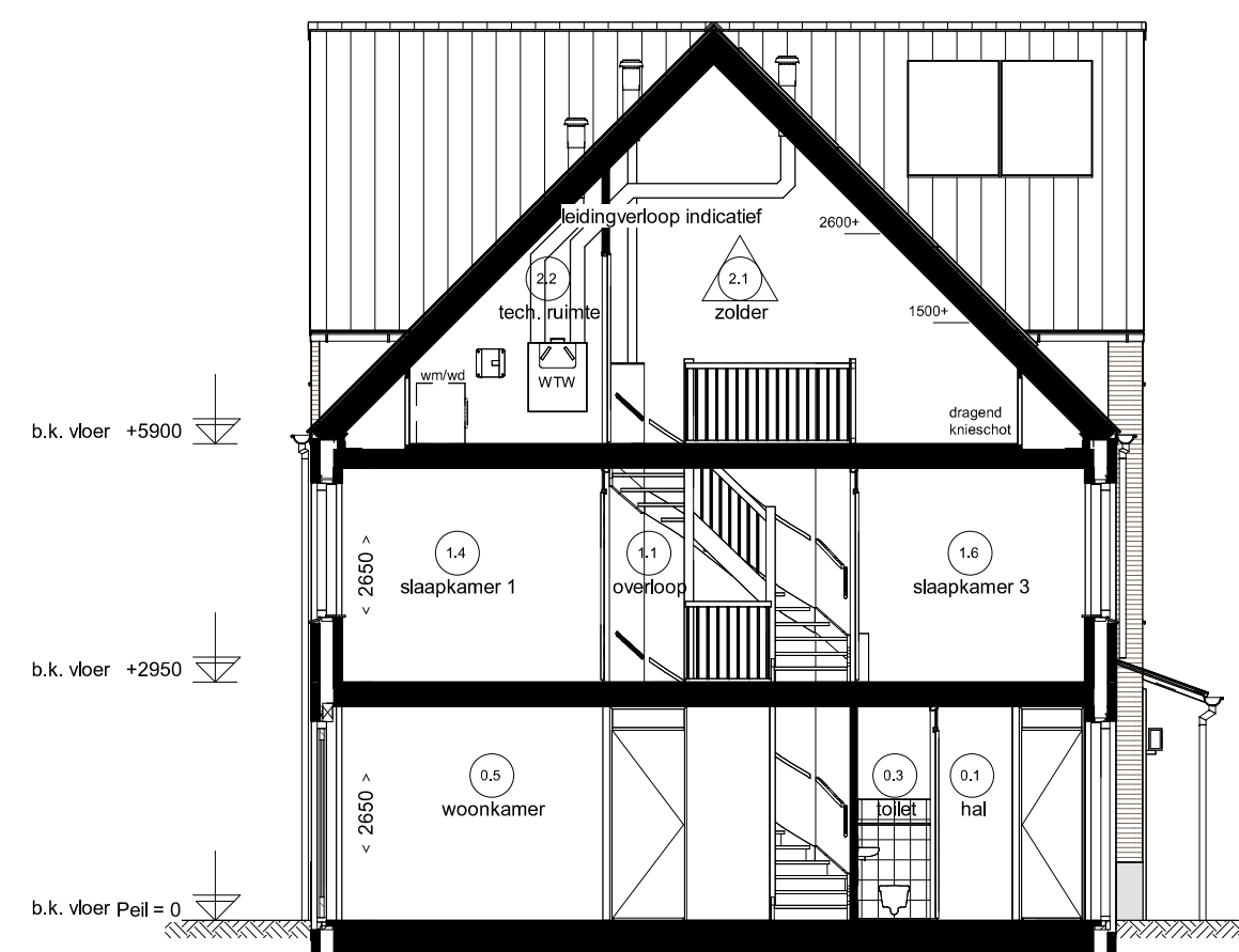
Doorsnede B02.1
