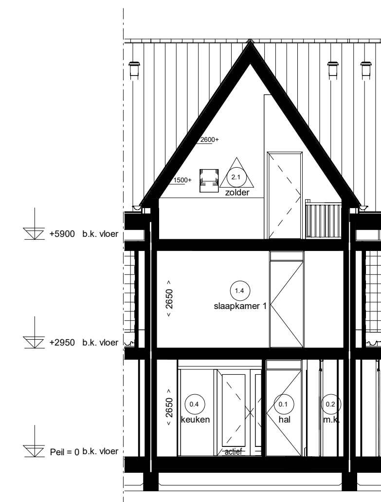
Doorsnede L10.3
