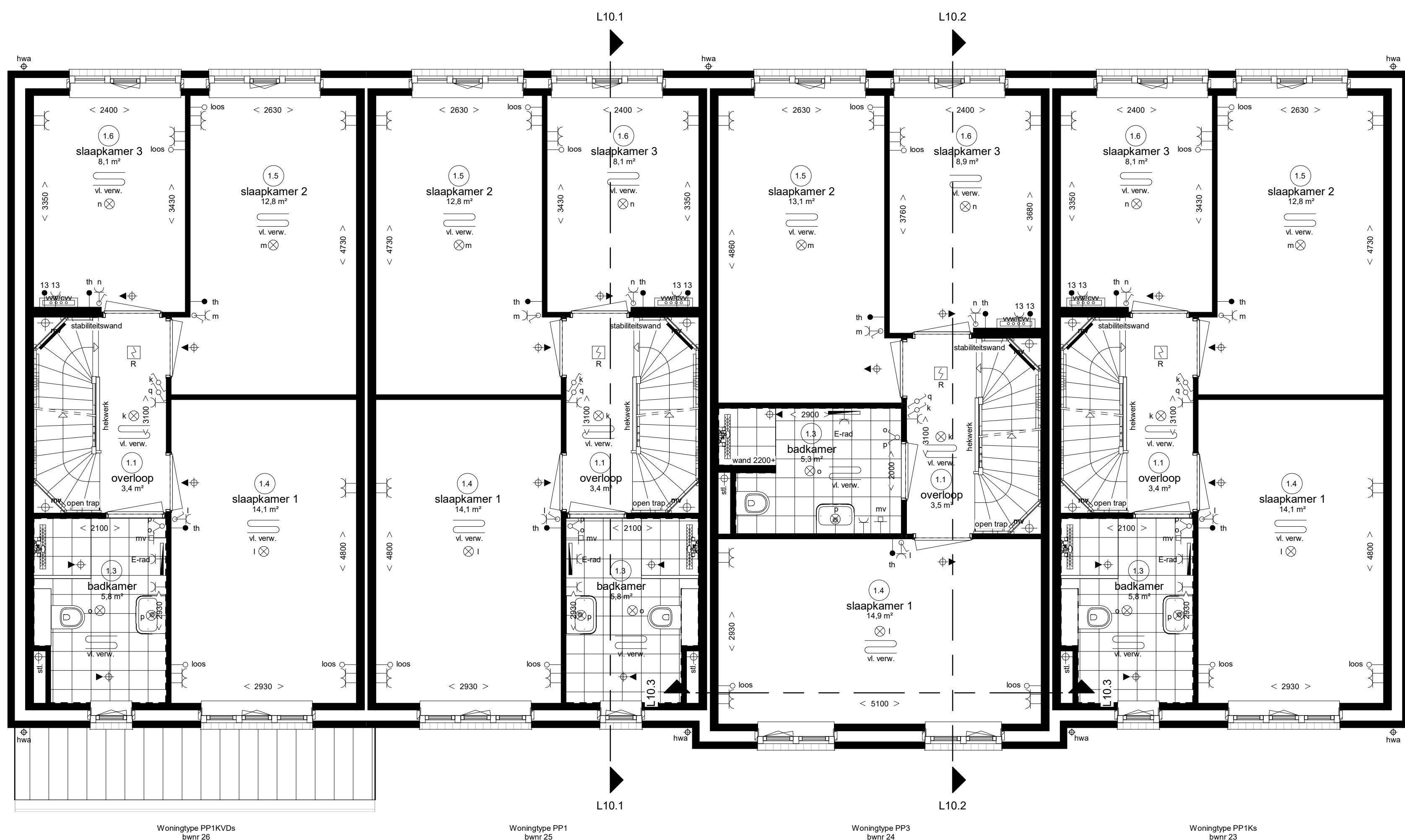
Eerste verdieping
