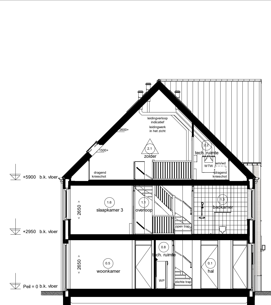
Doorsnede L10.1
