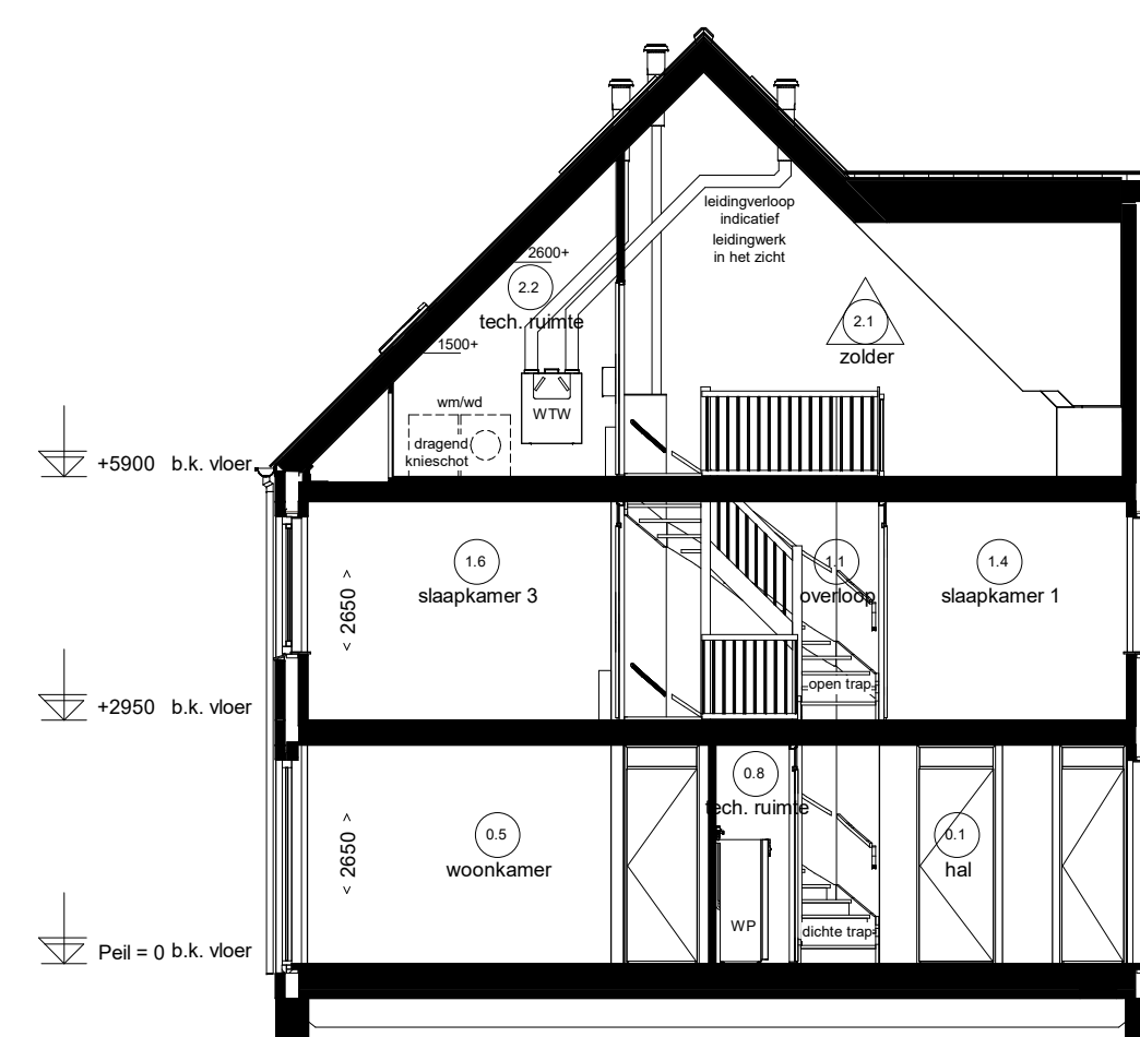
Doorsnede L10.2
