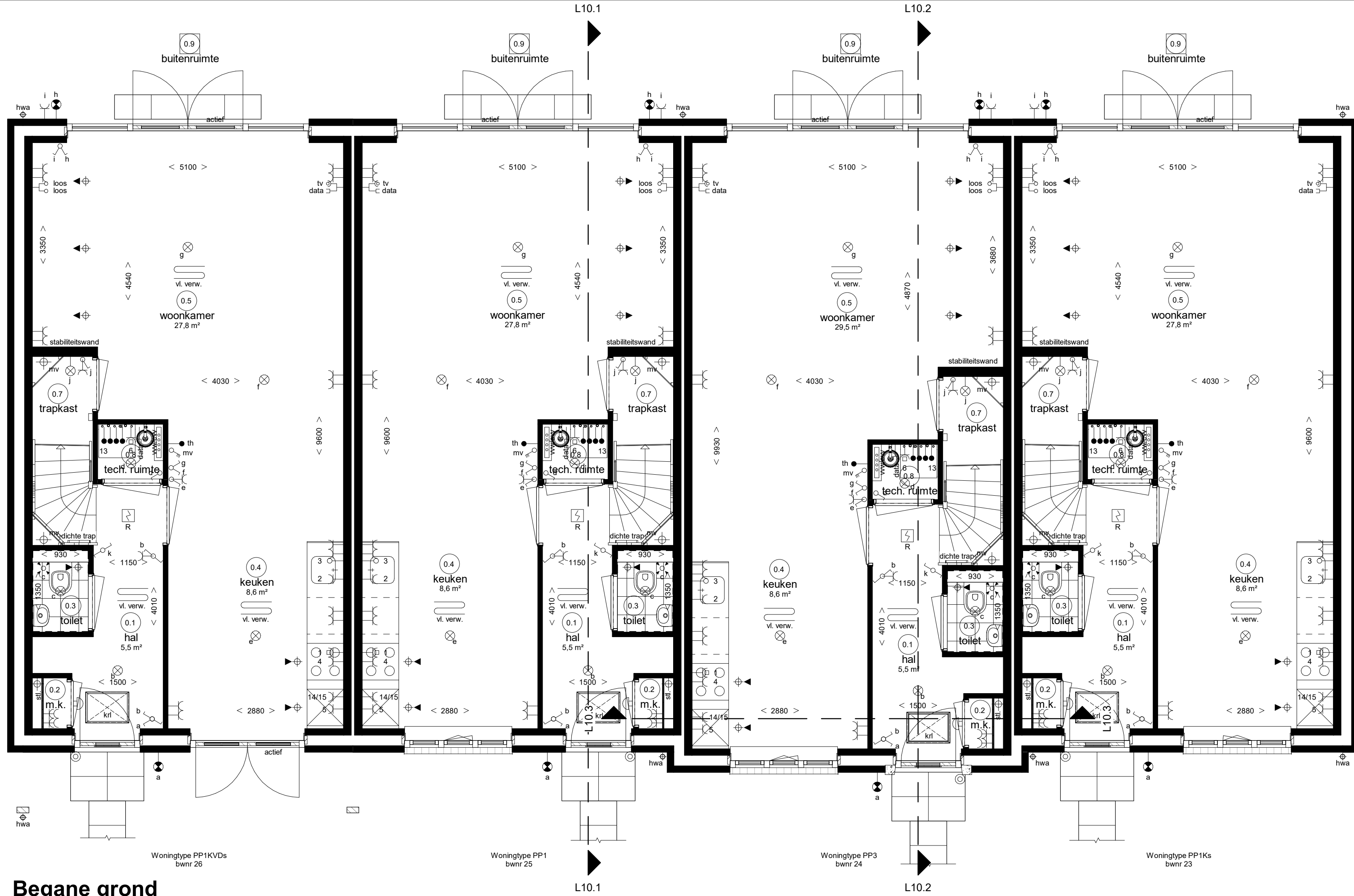
Begane grond
