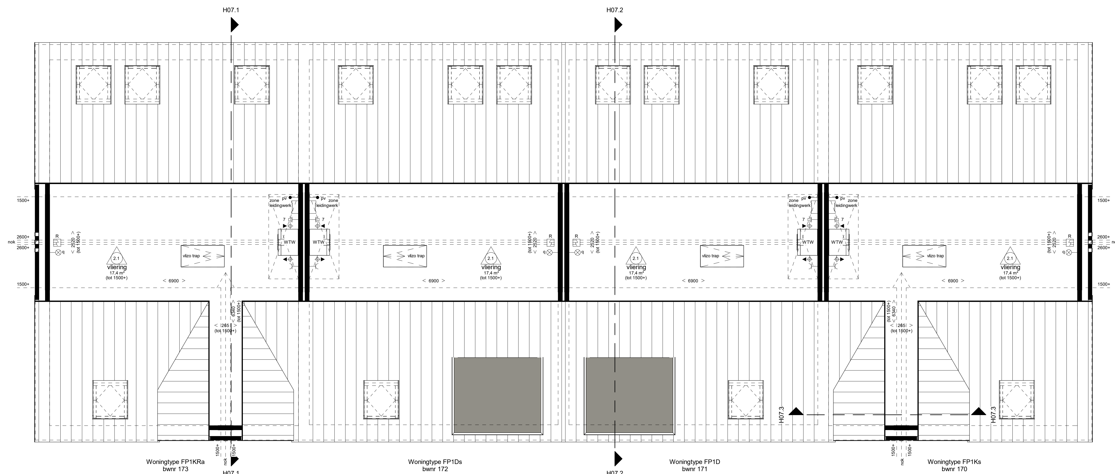
Tweede verdieping
