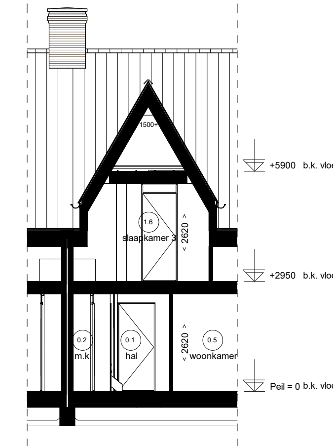
Doorsnede H07.3
