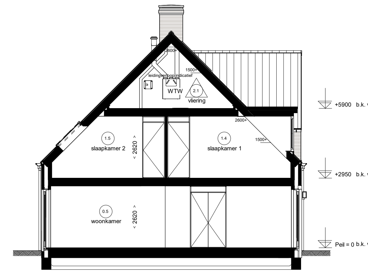
Doorsnede H07.2
