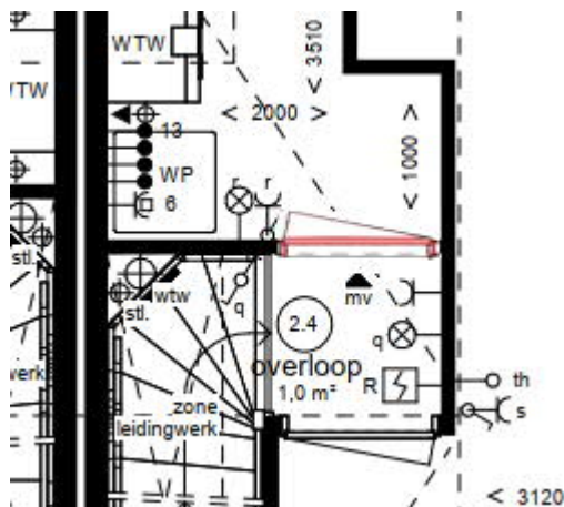
Fragment verkooptekening VT.B02-B; gewijzigde draairichting technische ruimte bwnr 367
