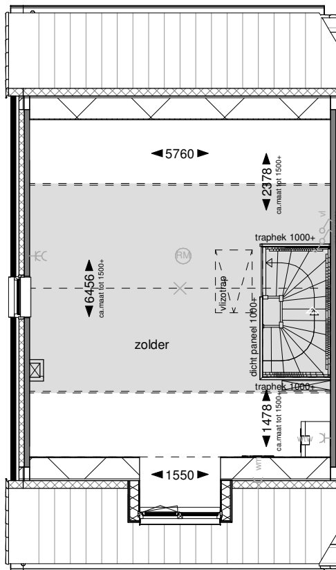
Tweede verdieping
