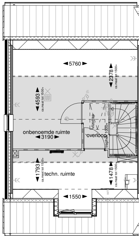
Tweede verdieping
