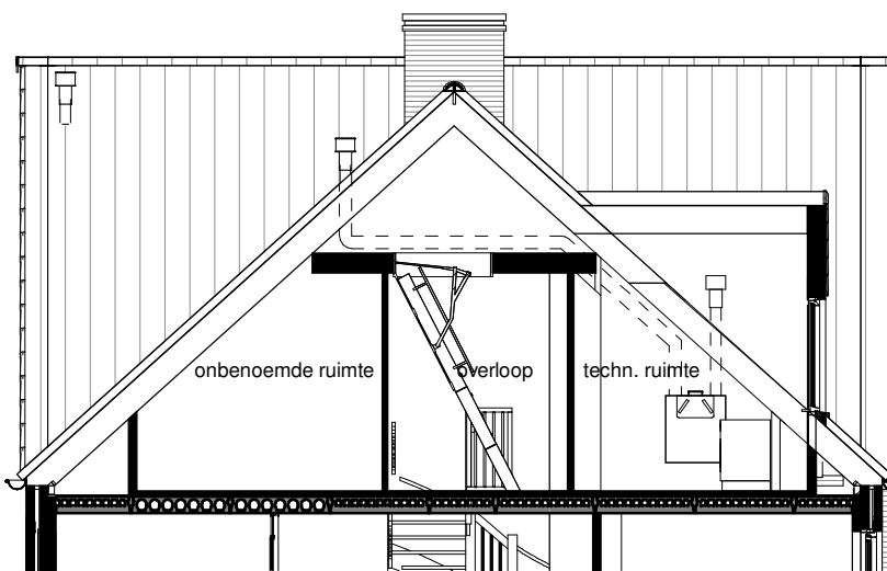
Doorsnede
