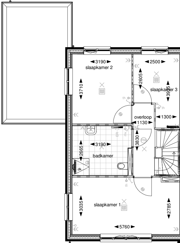
Eerste verdieping
