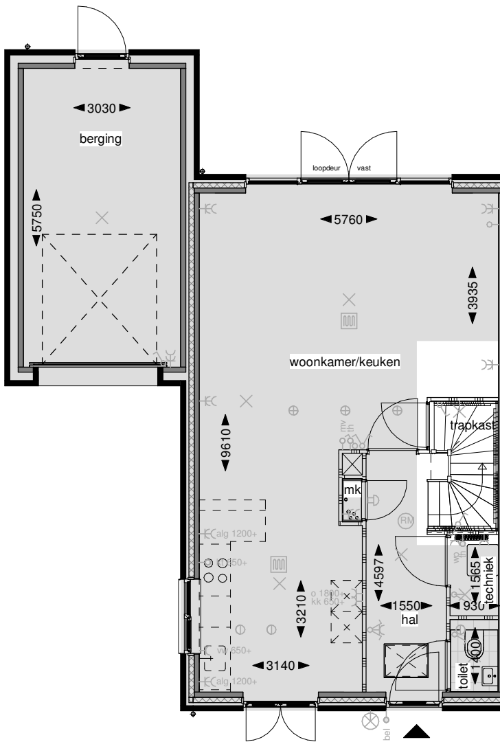
Begane grond
