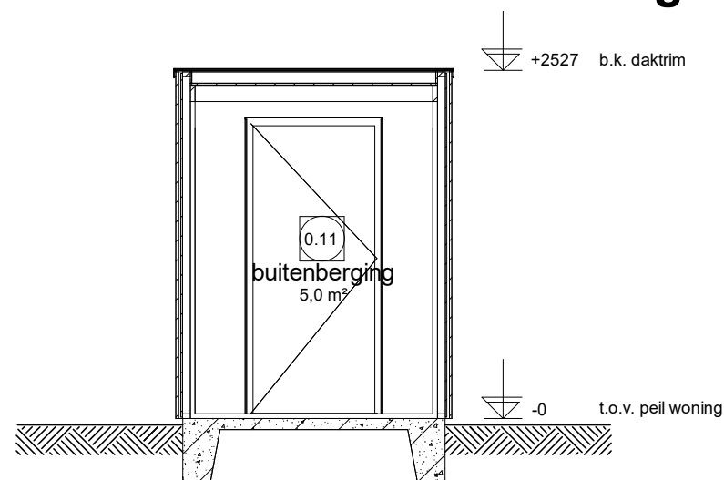
Doorsnede D1.1
