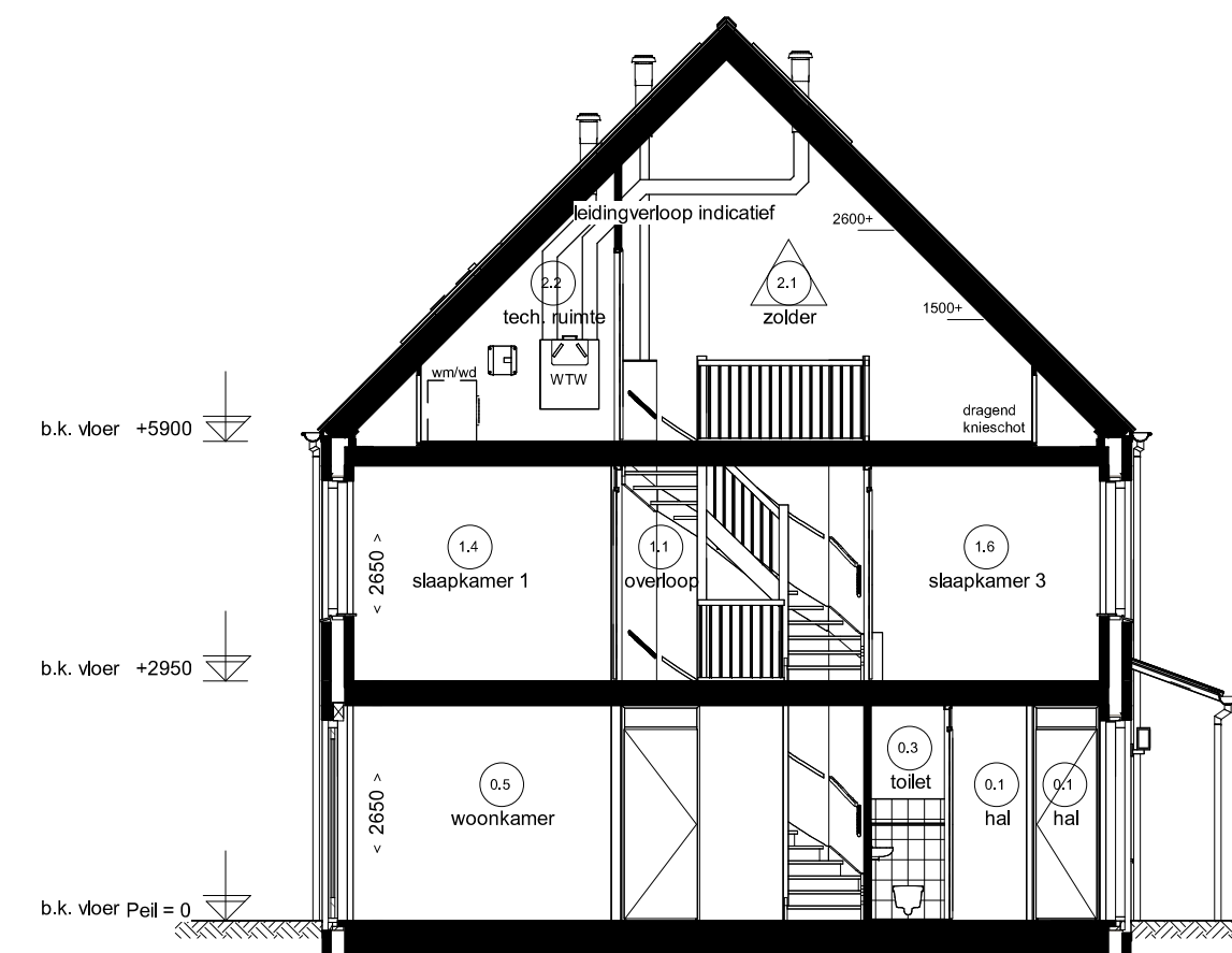
Doorsnede B04.1
