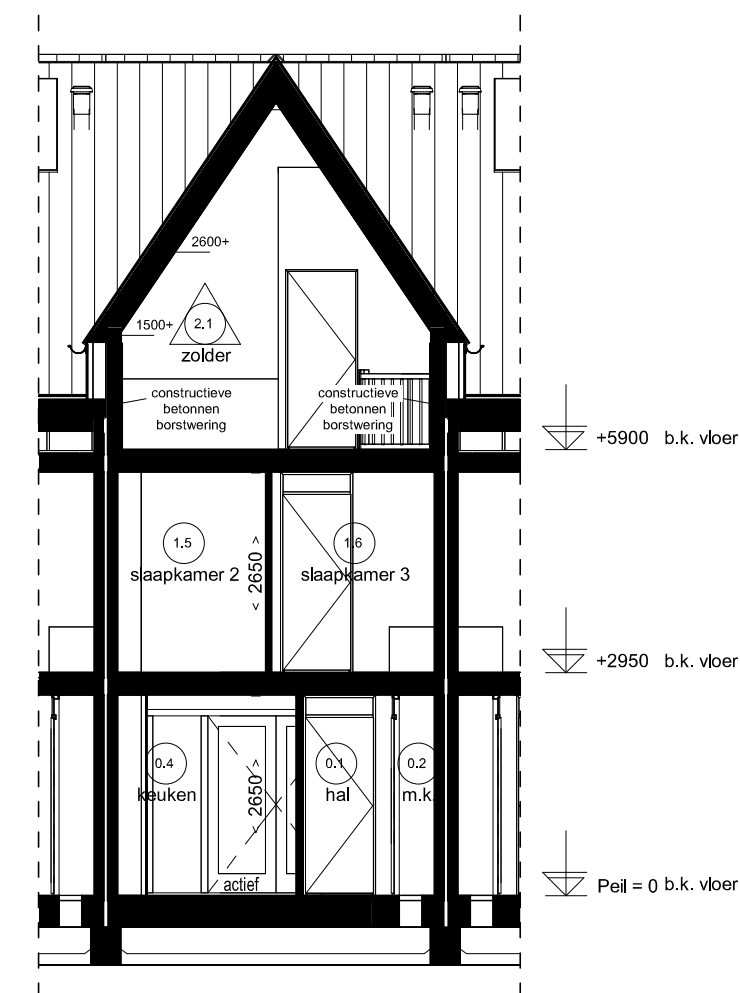
Doorsnede B04.2
