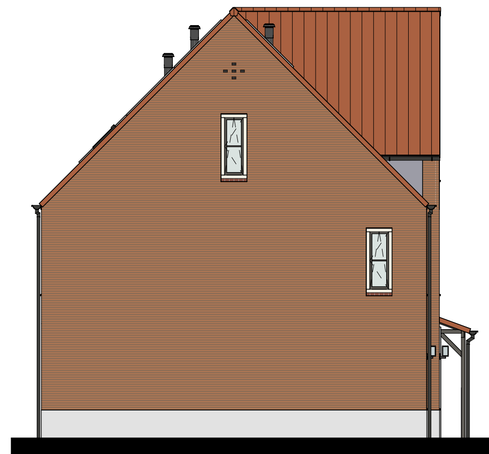
Linkergevel
