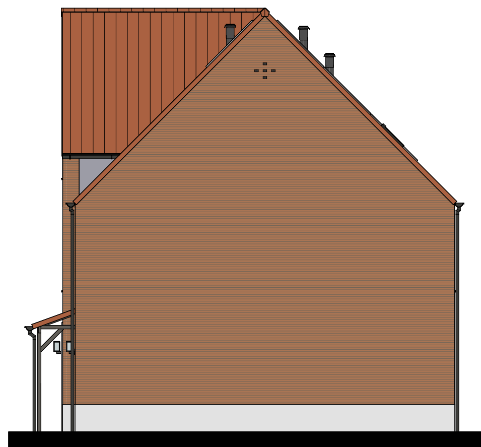
Rechtergevel
