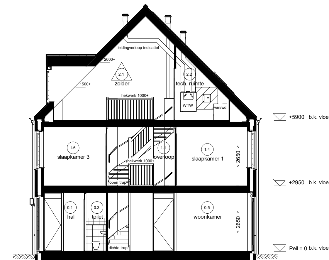
Doorsnede A12.1
