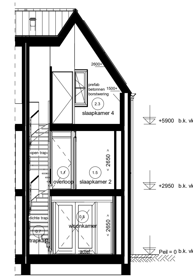
Doorsnede A12.3
