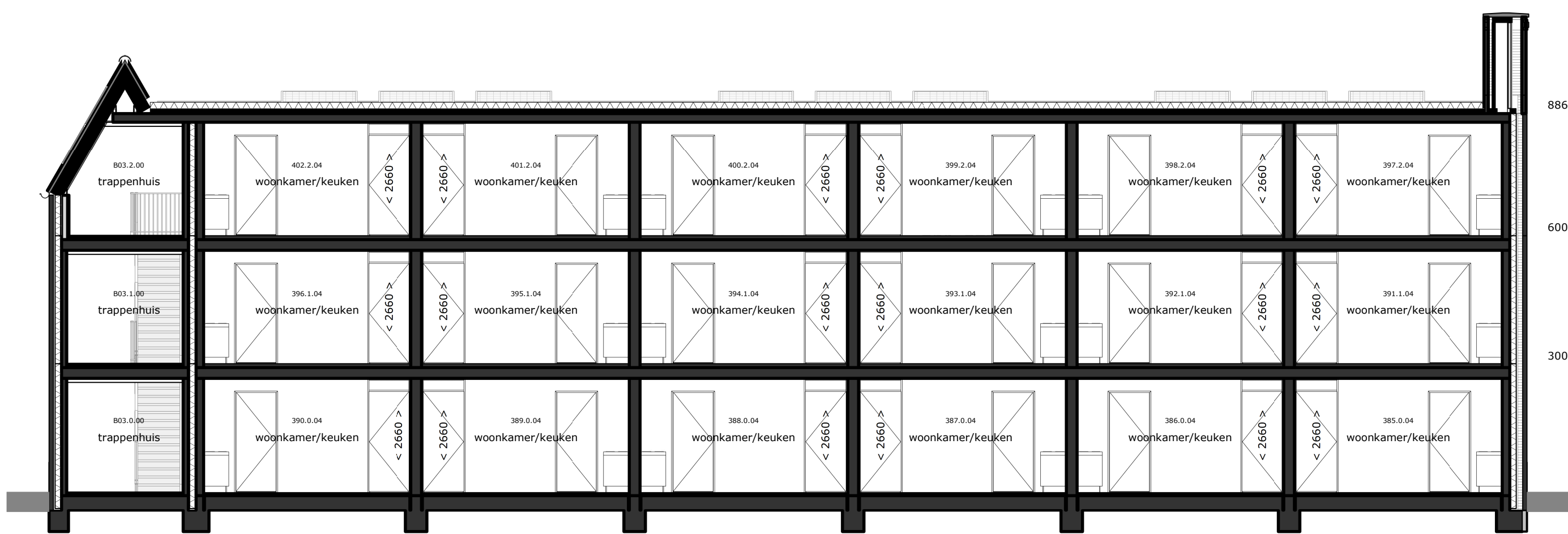
doorsnede 1-1
