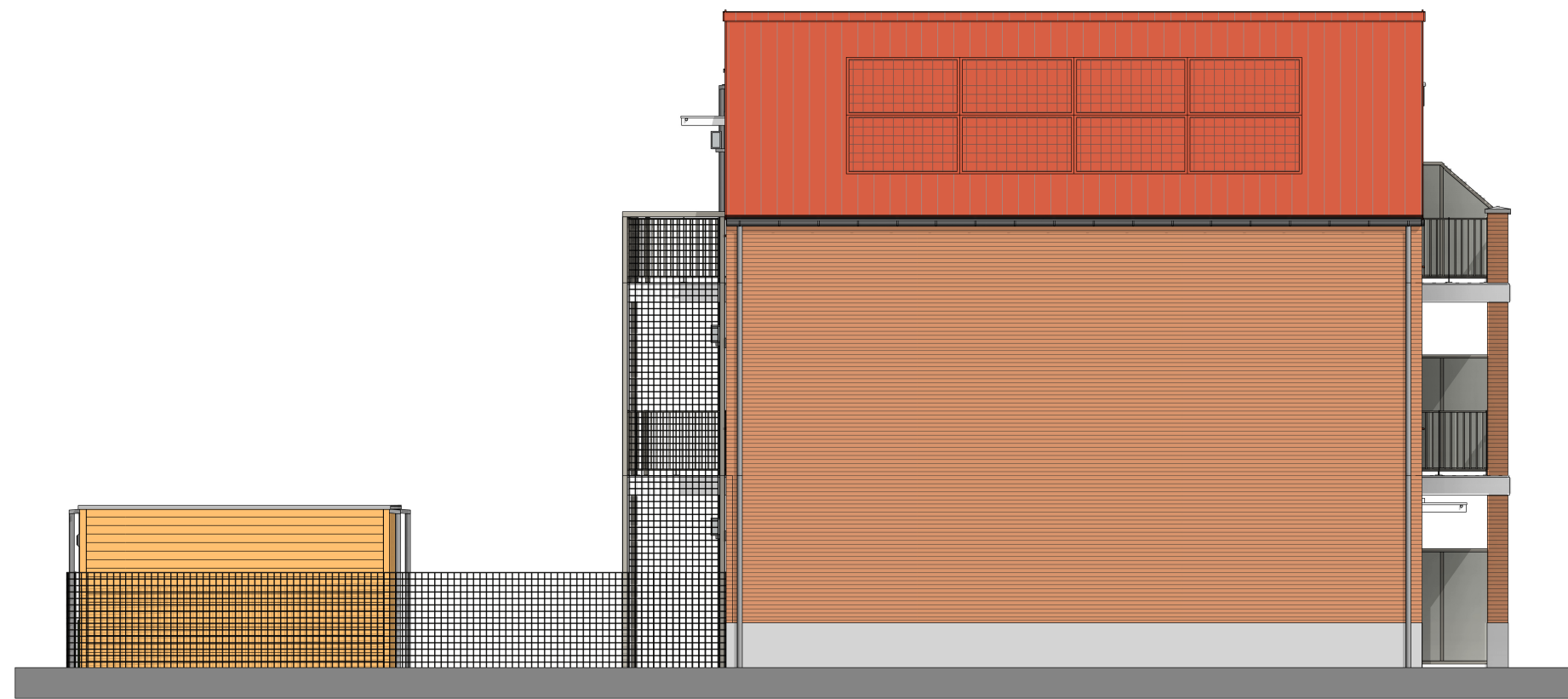
linkergevel (oriëntatie: zuid)
