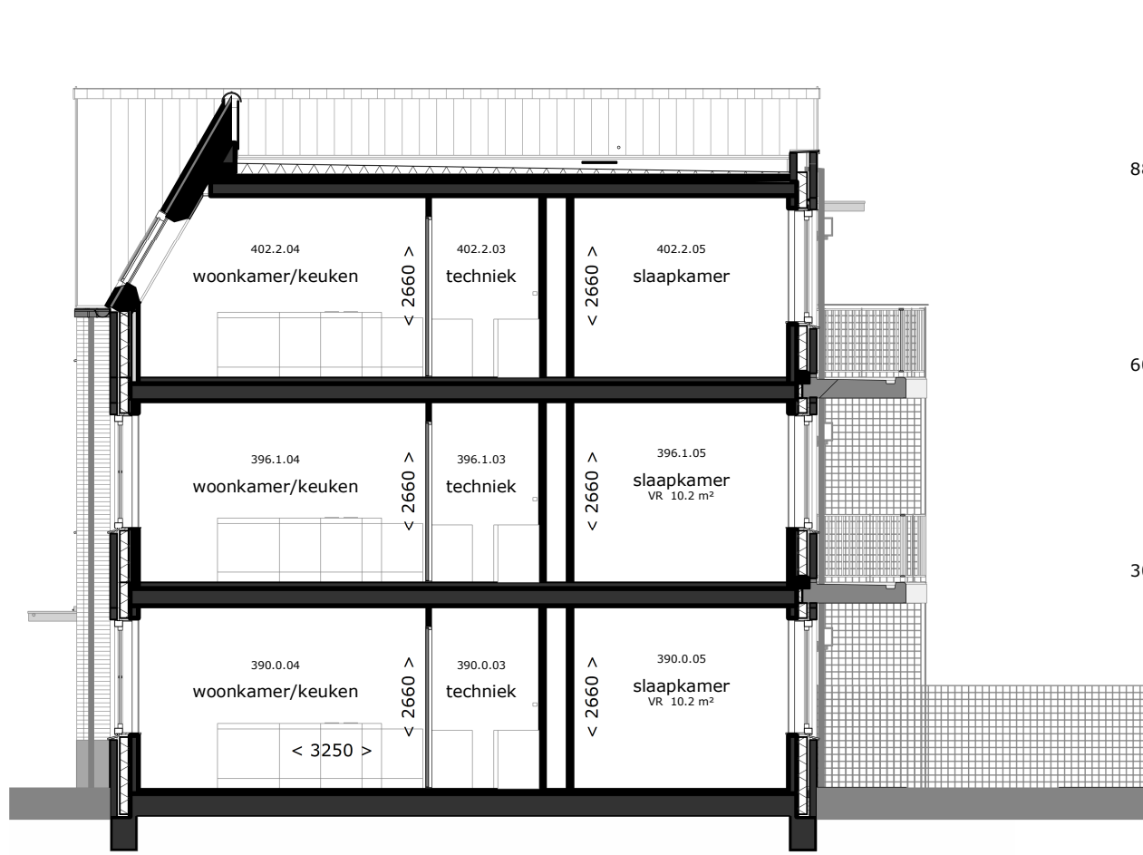
doorsnede B-B
