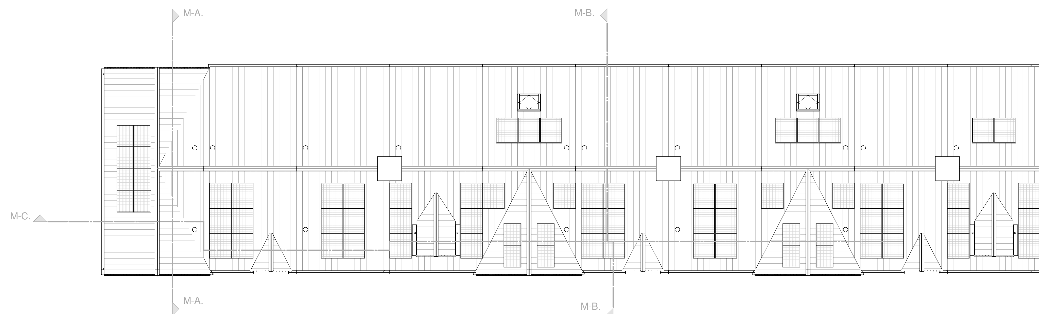
Dakaanzicht
