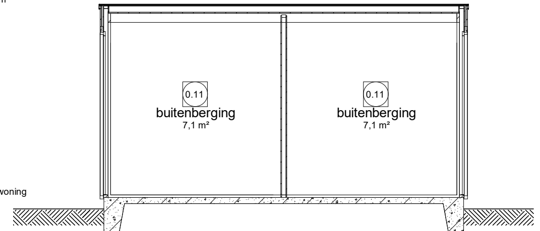
Doorsnede D4.2
