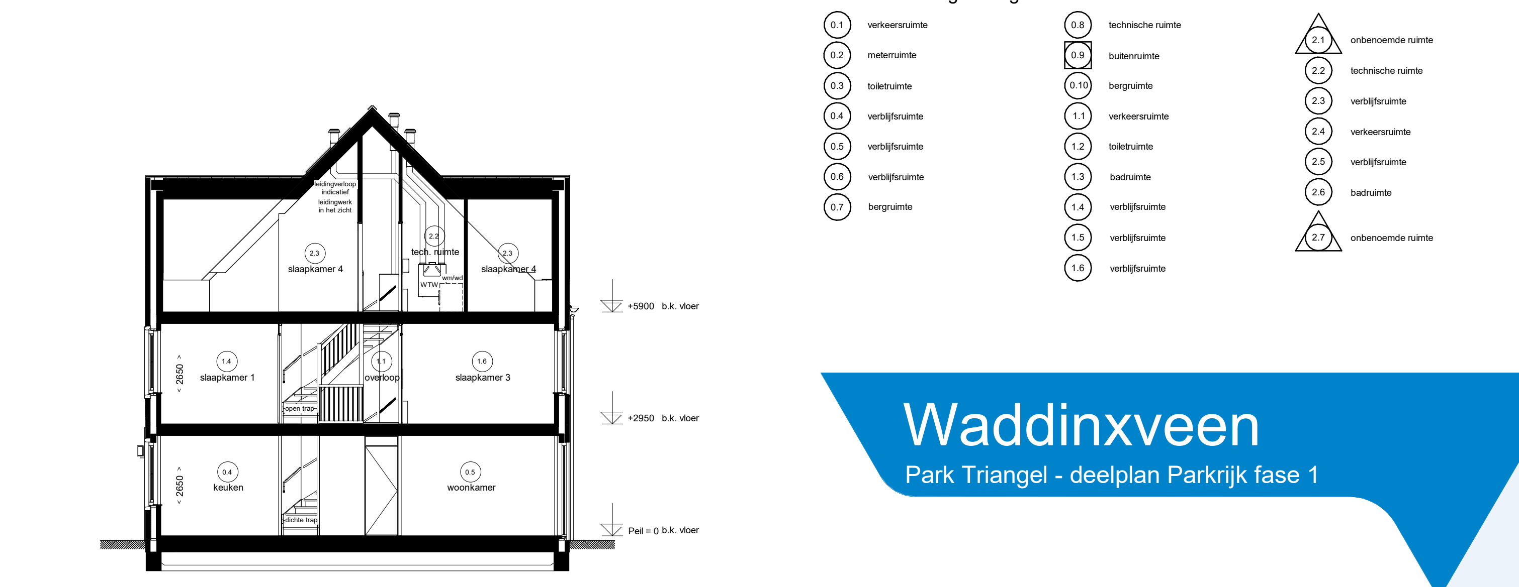
Doorsnede L08.2
