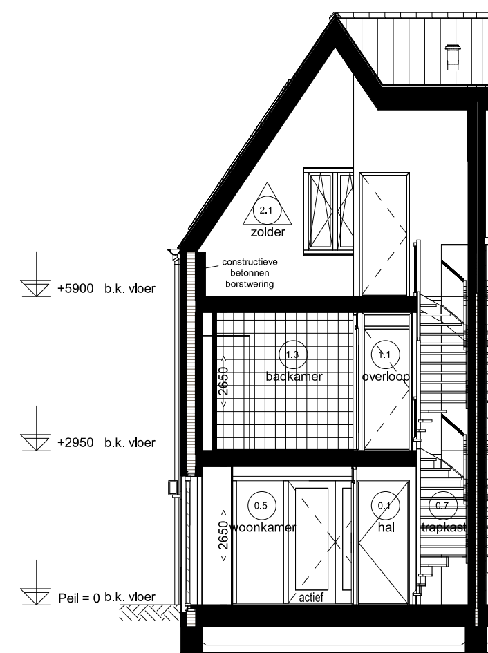
Doorsnede B05.2
