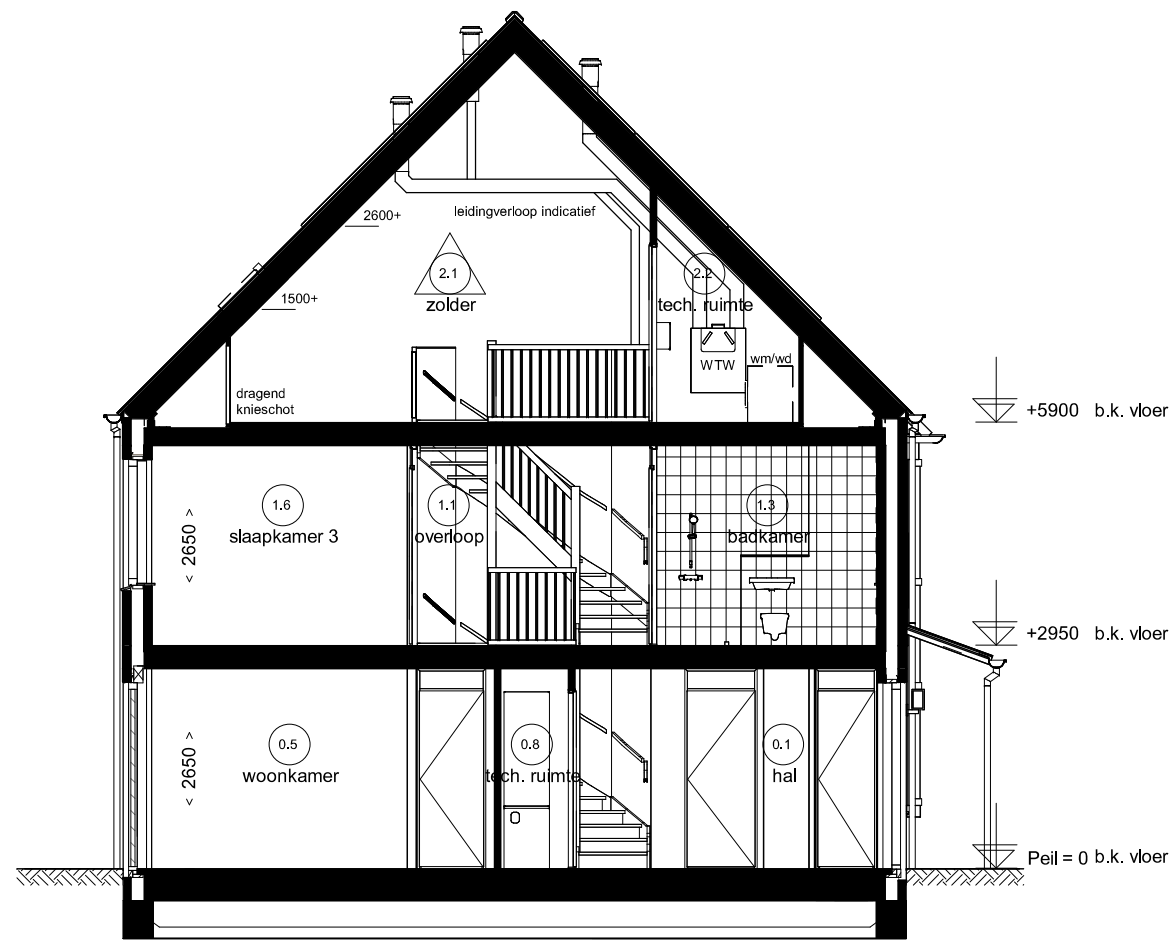
Doorsnede B05.1
