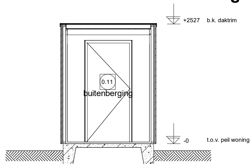
Doorsnede D1.1
