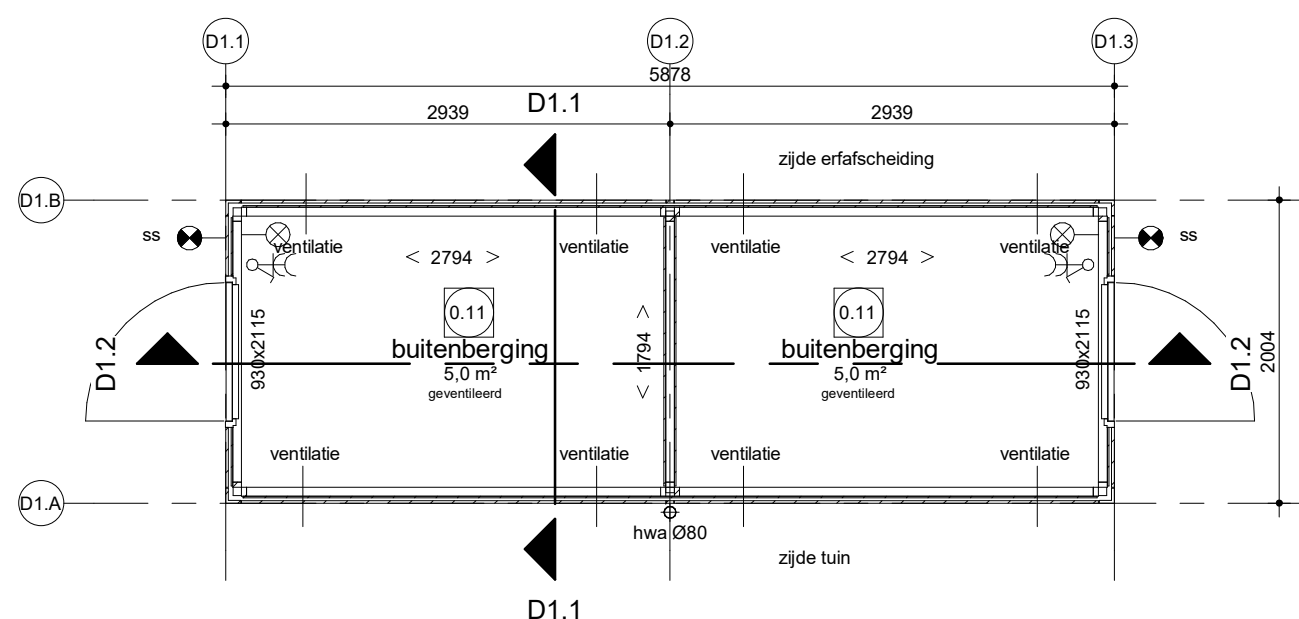
Begane grond
