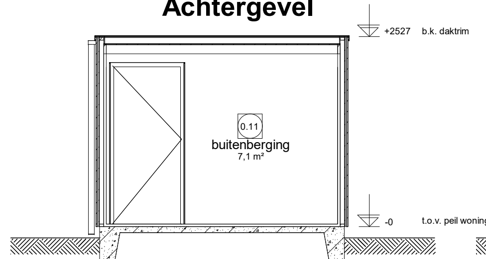
Doorsnede D4.1
