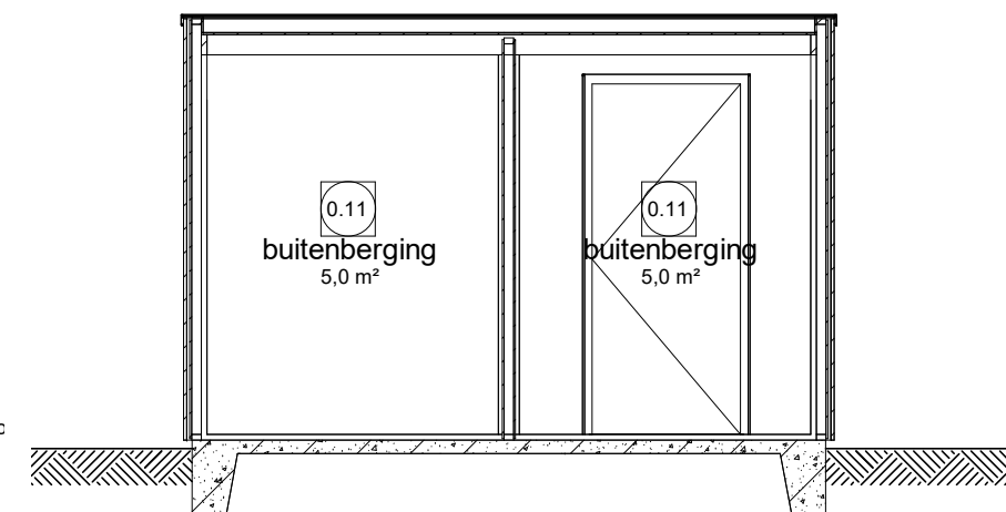
Doorsnede D5.2
