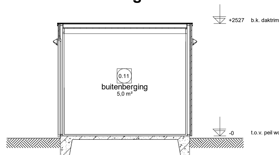
Doorsnede D5.1
