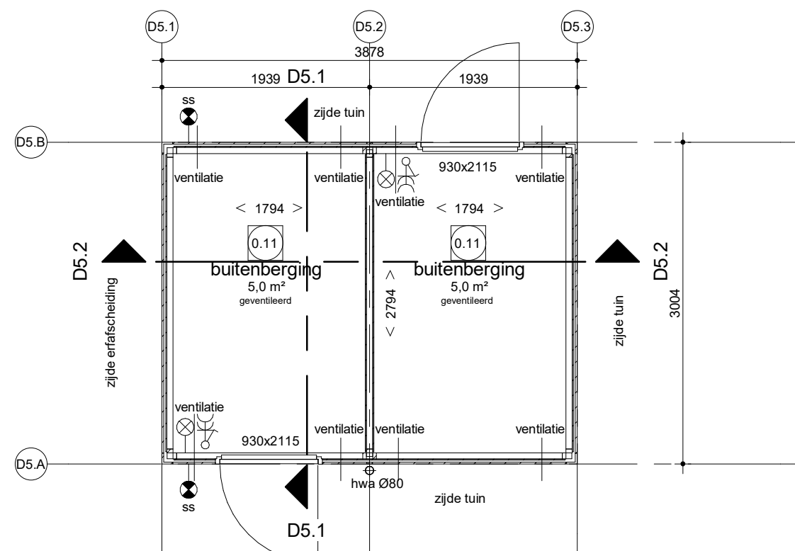
Begane grond
