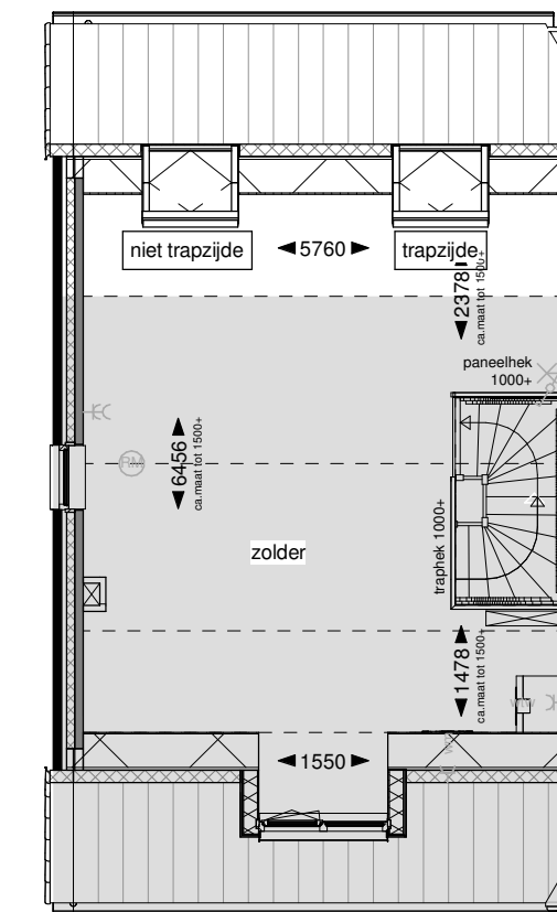
Tweede verdieping
