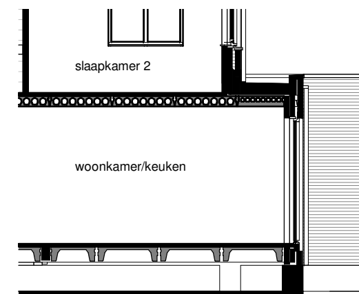
Doorsnede
