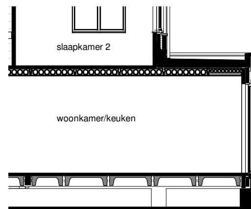
Doorsnede
