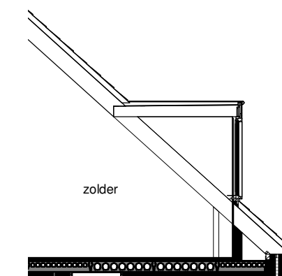
Doorsnede
