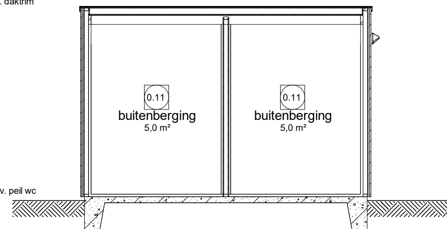
Doorsnede D6.2
