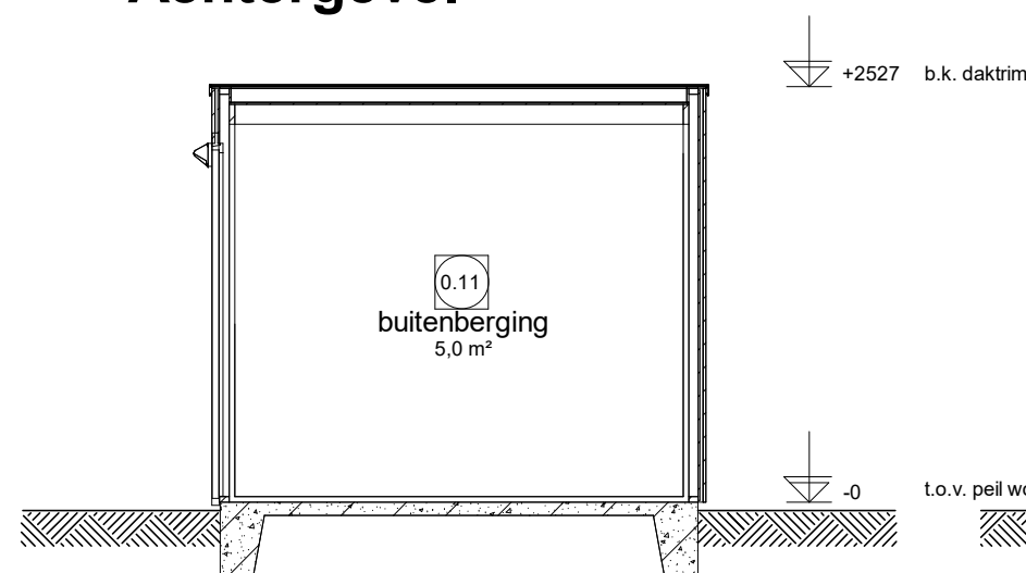
Doorsnede D6.1
