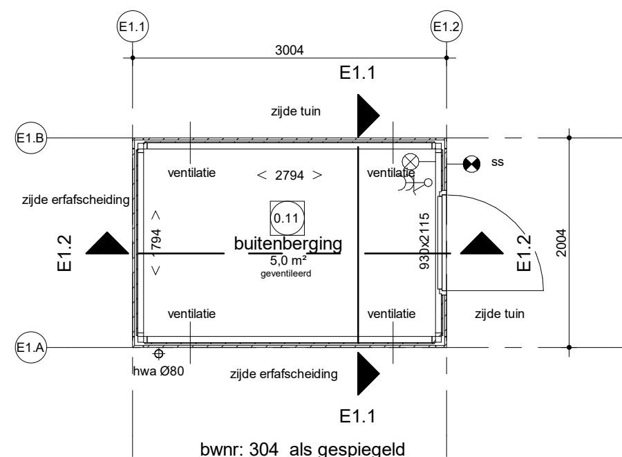
Begane grond
