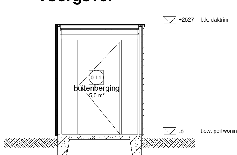
Doorsnede E1.1
