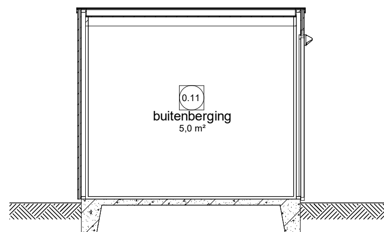
Doorsnede E1.2
