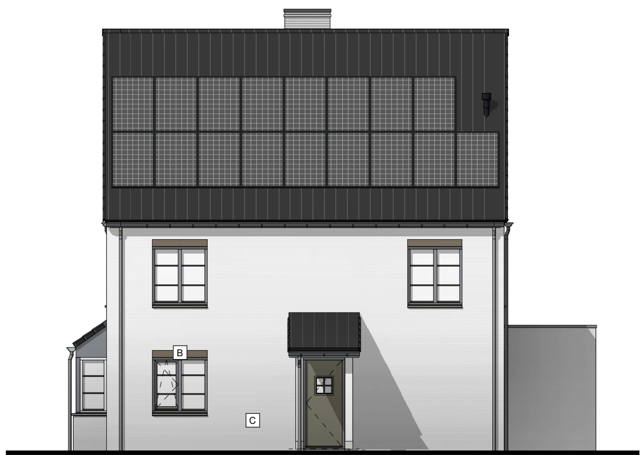
Type: Z.60.10.2 bwnr: 36 Rechter zijgevel
