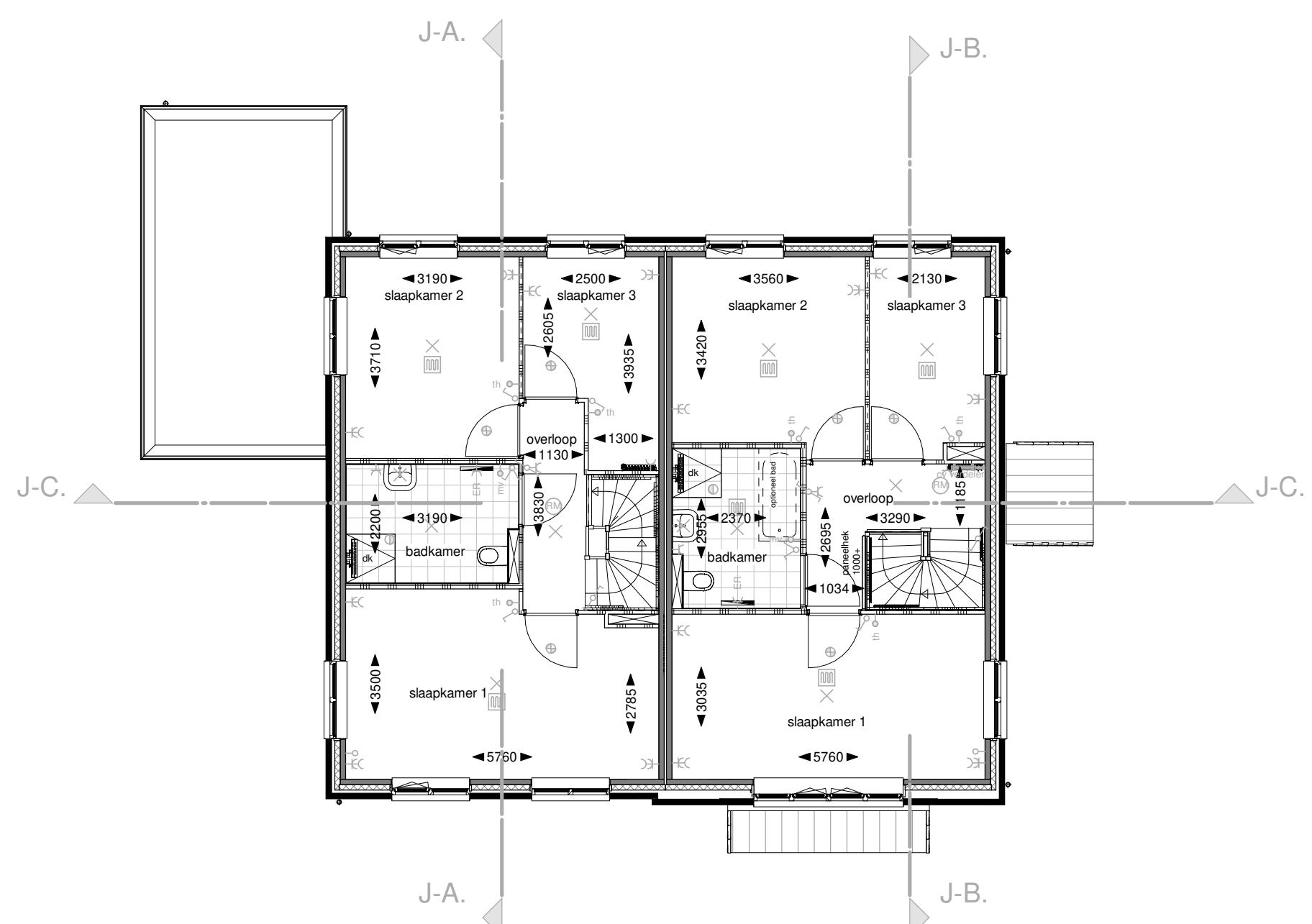
Type: V.60.10 bwnr: 37 Type: Z.60.10.2 bwnr: 36 Eerste verdieping
