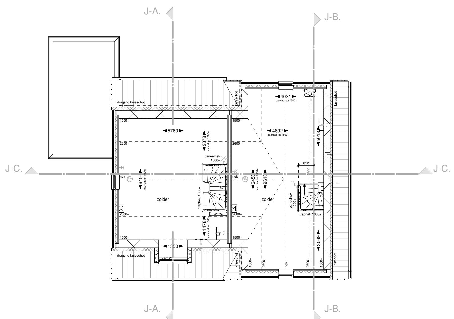
Type: V.60.10 bwnr: 37 Type: Z.60.10.2 bwnr: 36 Tweede verdieping
