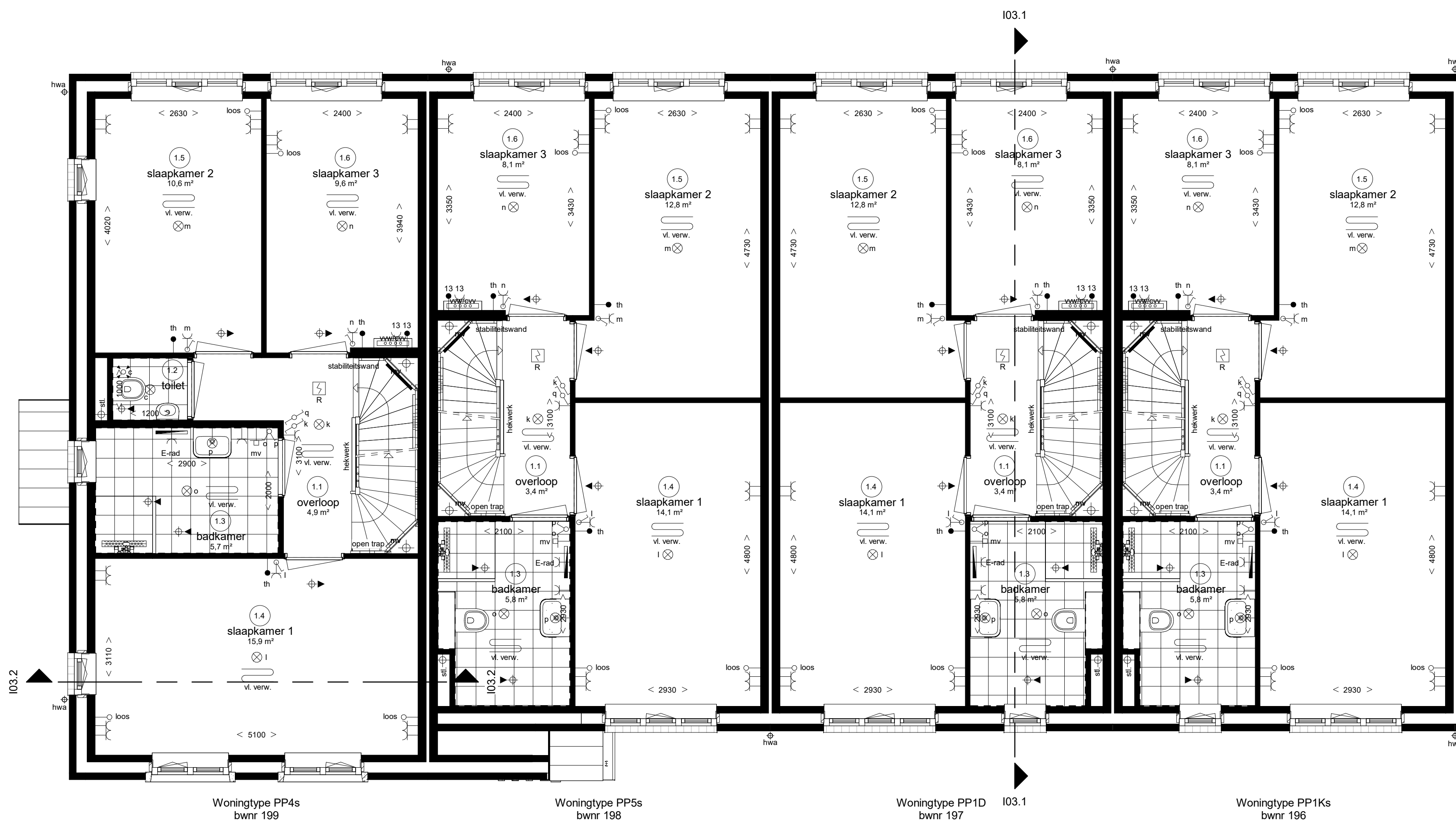
Eerste verdieping
