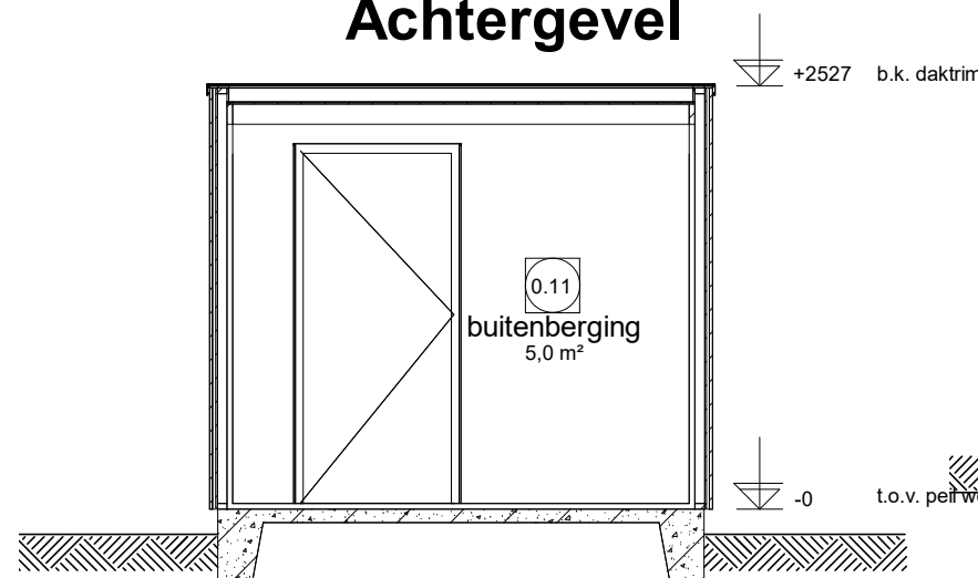
Doorsnede D4.1
