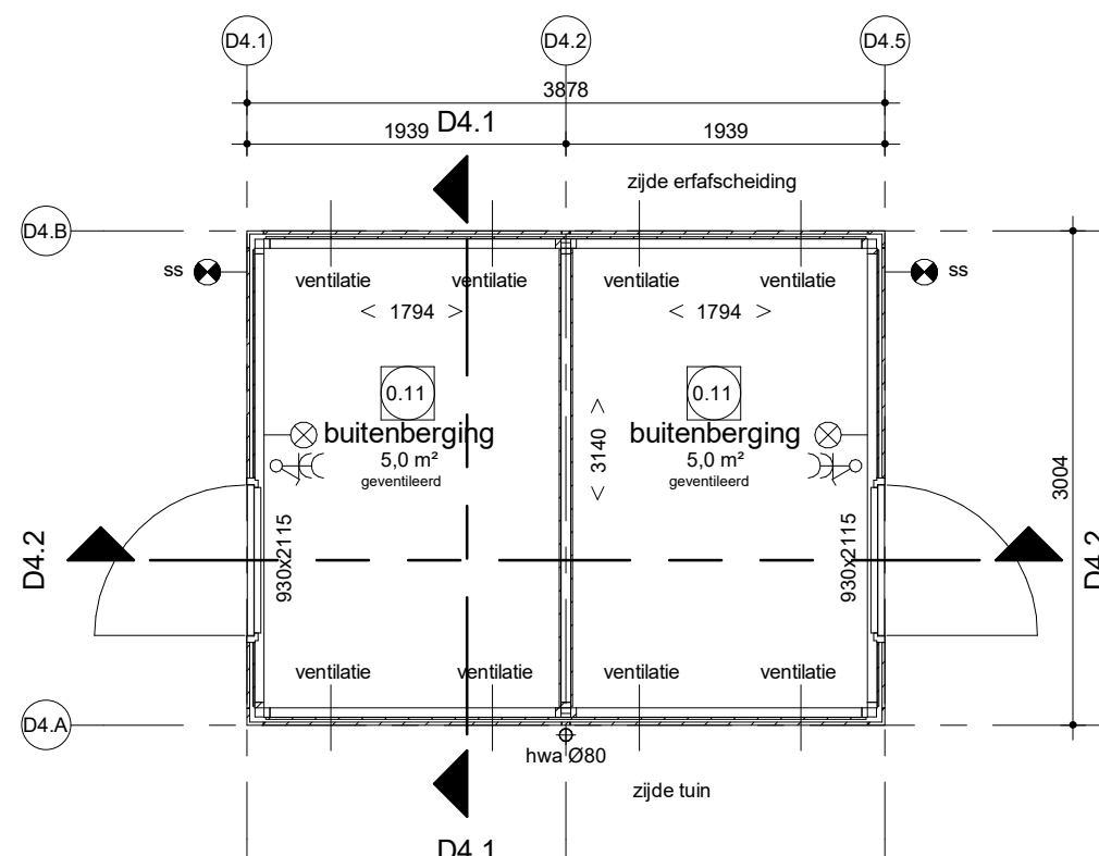
Begane grond
