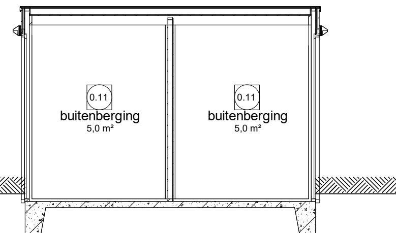
Doorsnede D4.2
