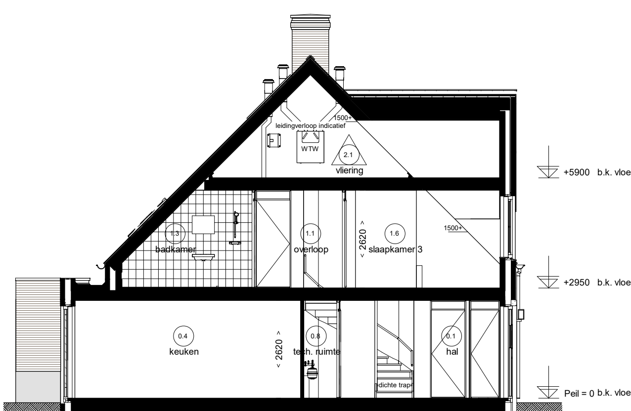
Doorsnede J04.4
