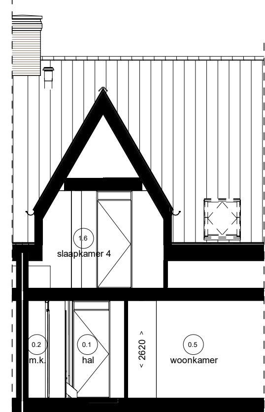
Doorsnede J04.6
