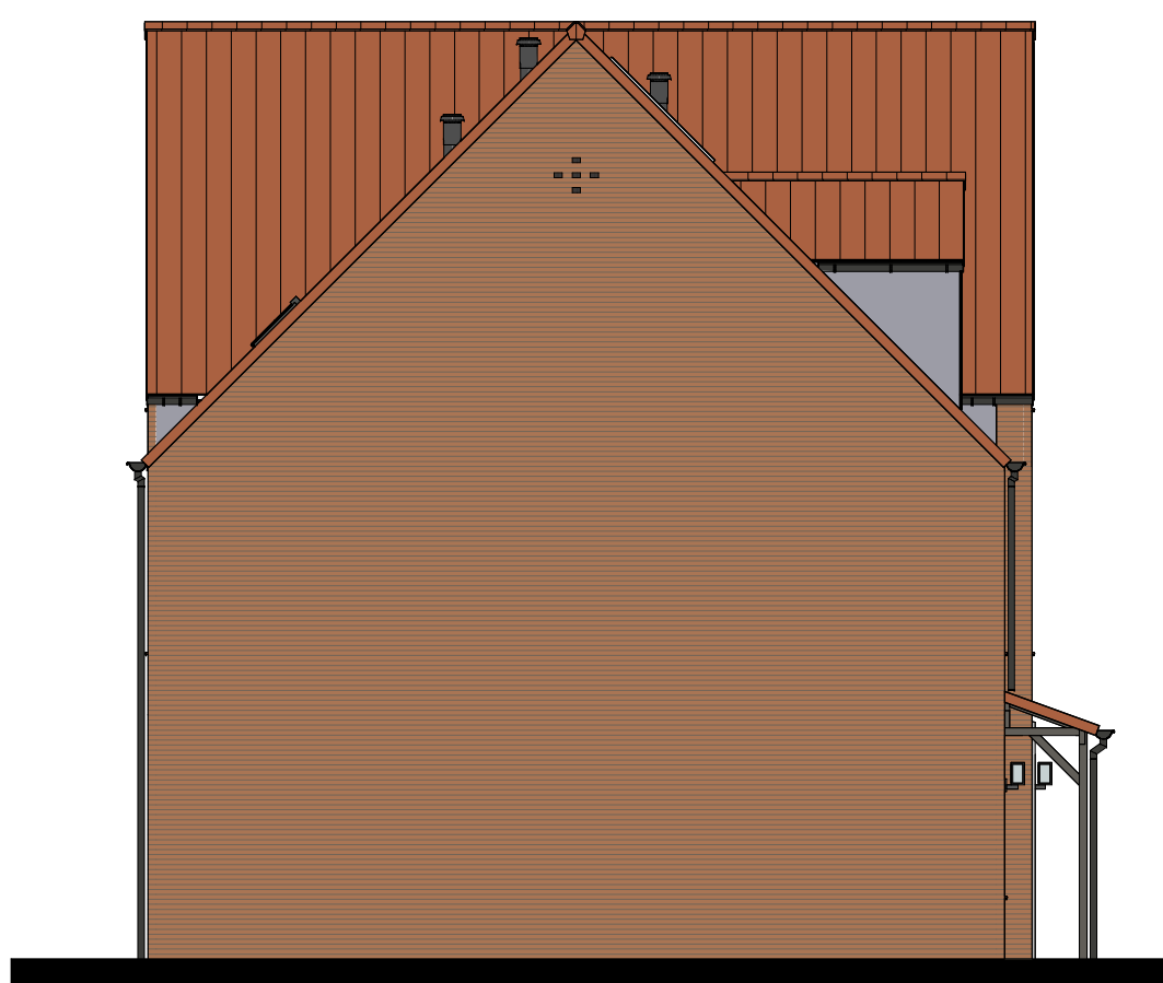
Woningtype P1K bwnr 122
