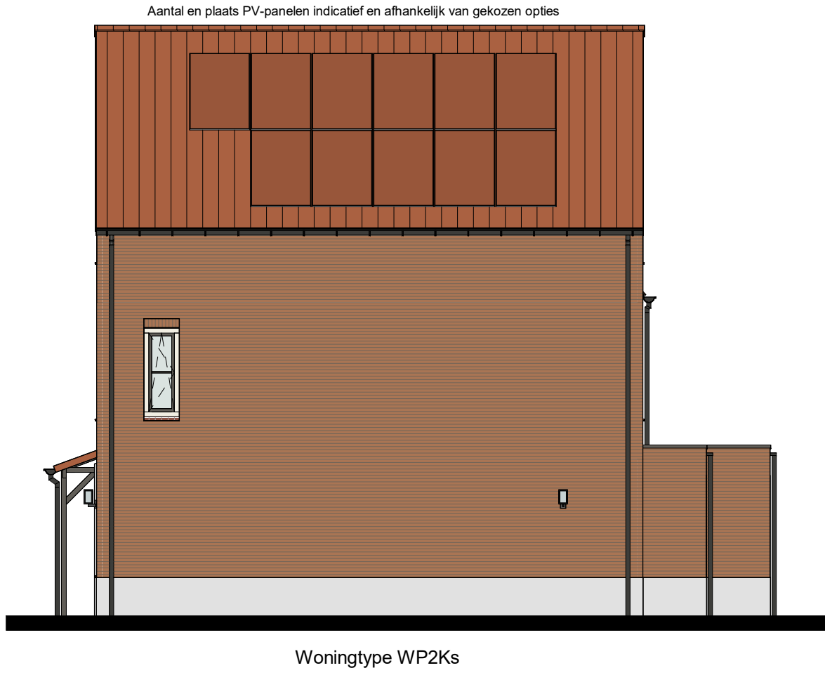
rechtergevel
