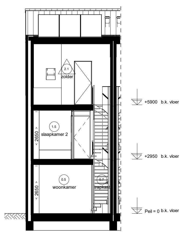
Doorsnede F10.7
