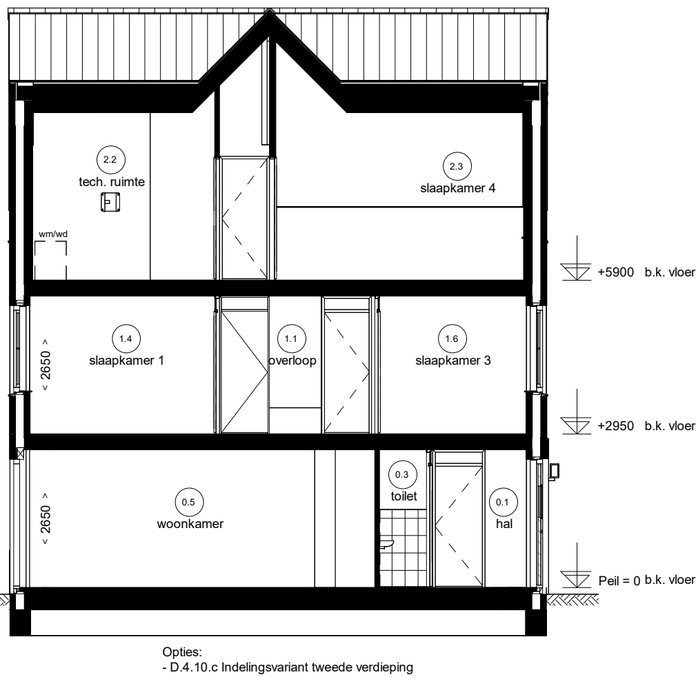
Doorsnede F10.6
