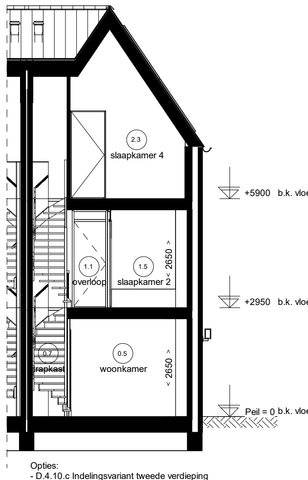
Doorsnede F10.8
