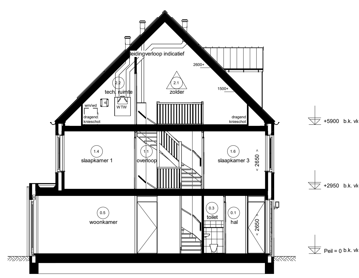
Doorsnede F10.5
