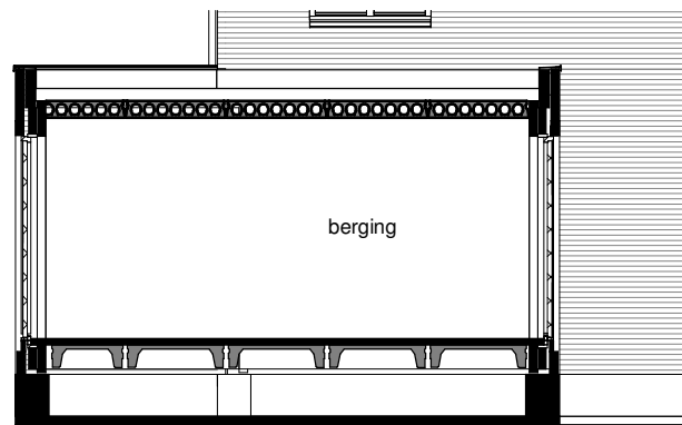
Fragment doorsnede
