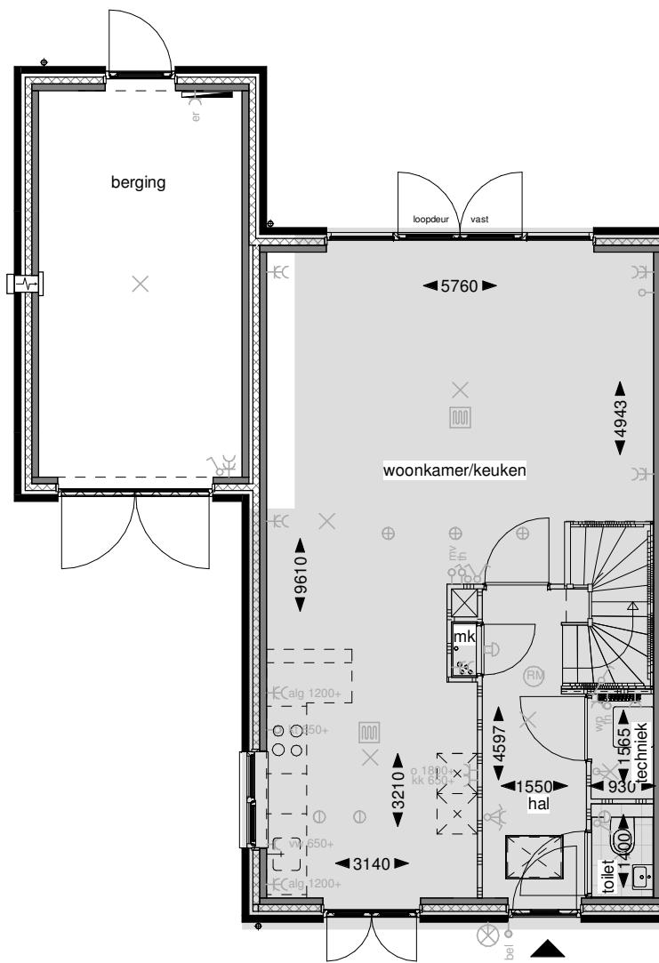
Begane grond
