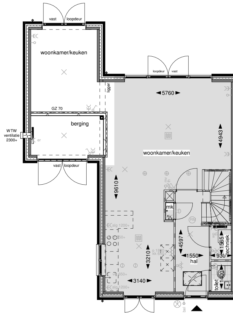
Begane grond
