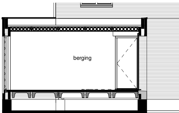
Fragment doorsnede
