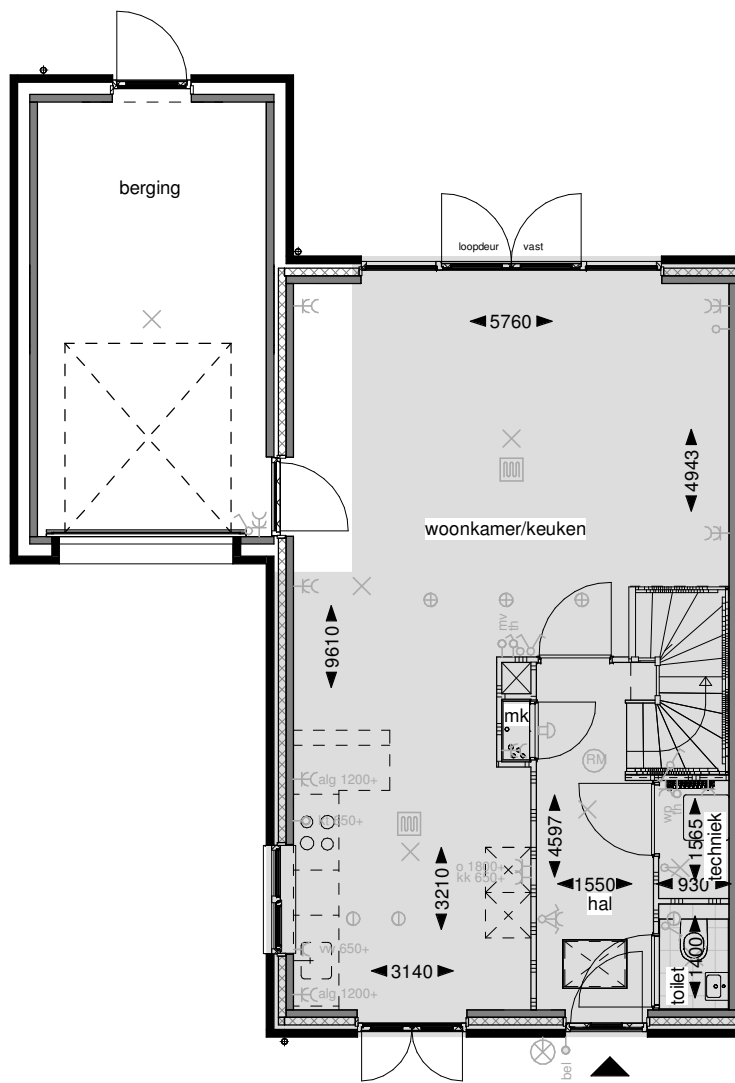
Begane grond
