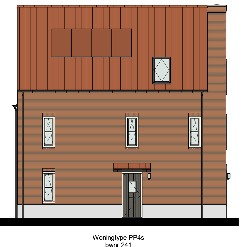
Linkergevel
