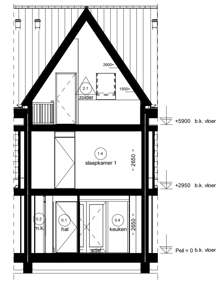
Doorsnede D04.3
