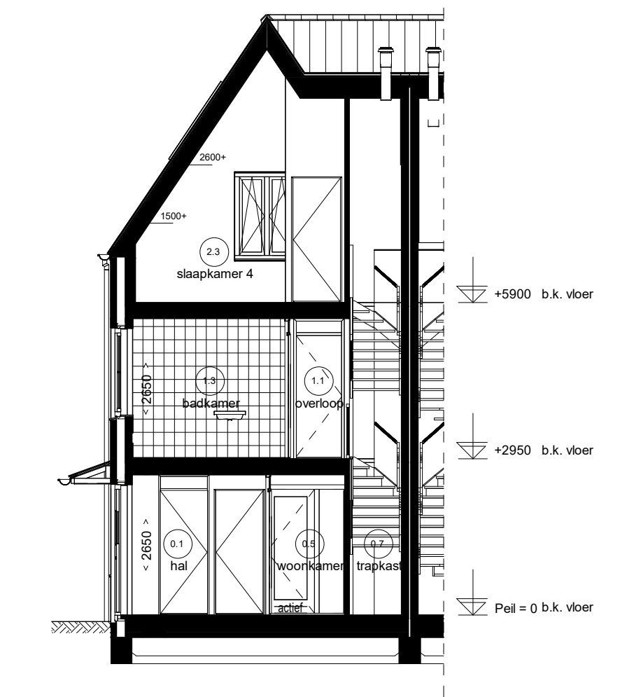
Doorsnede D04.2
