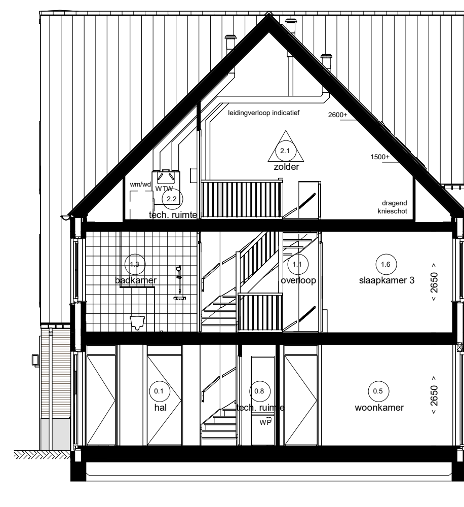
Doorsnede D04.1
