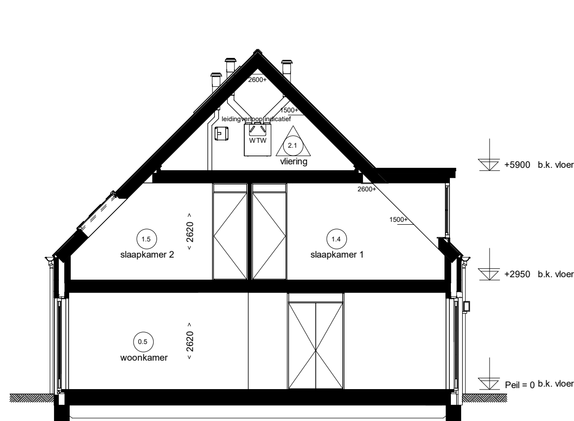
Doorsnede H09.2
