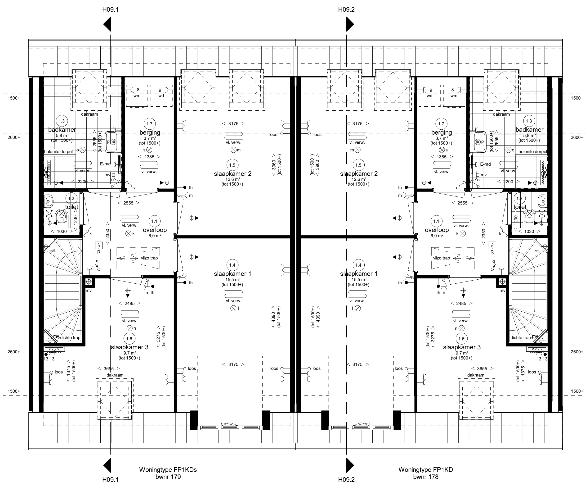
Eerste verdieping
