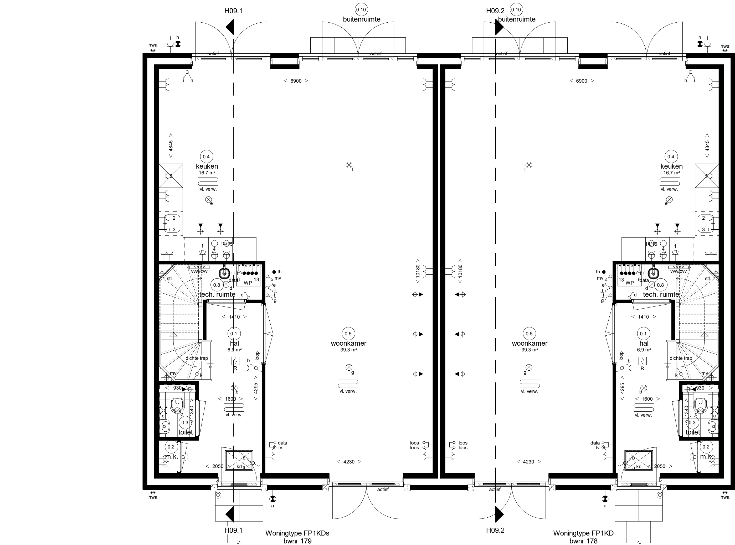
Begane grond
