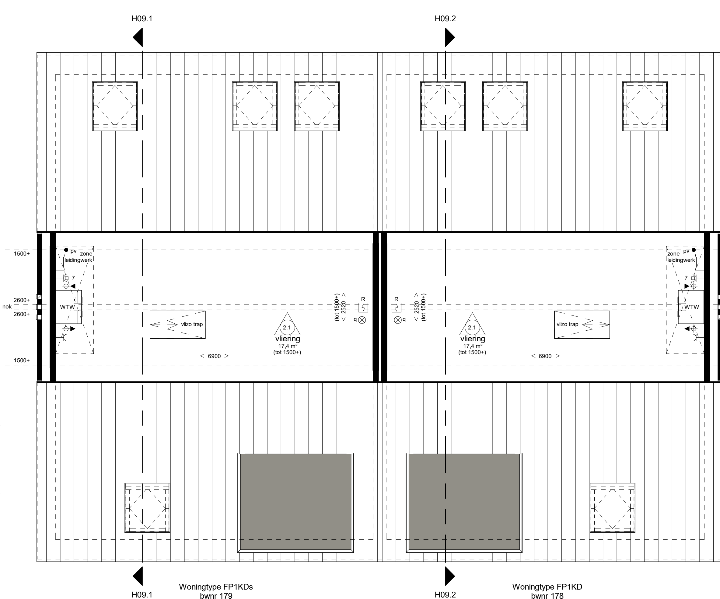
Tweede verdieping
