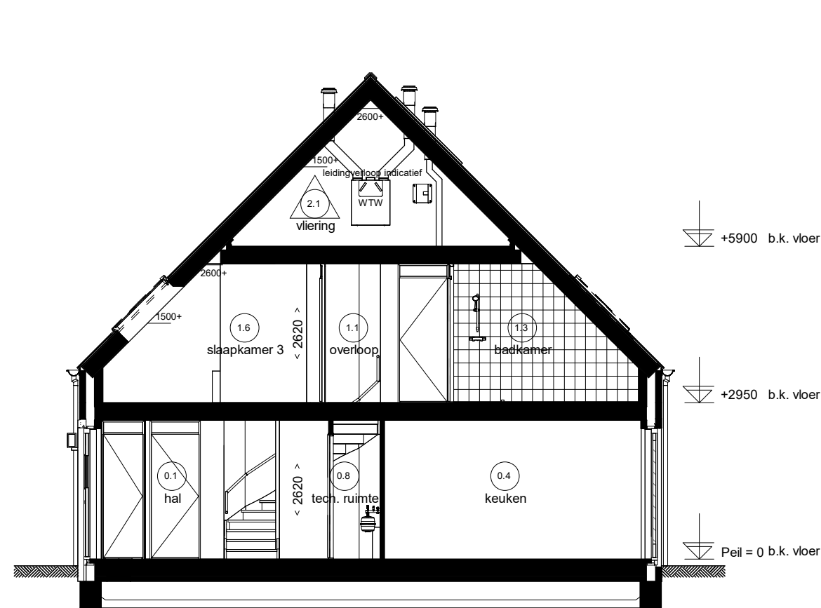
Doorsnede H09.1
