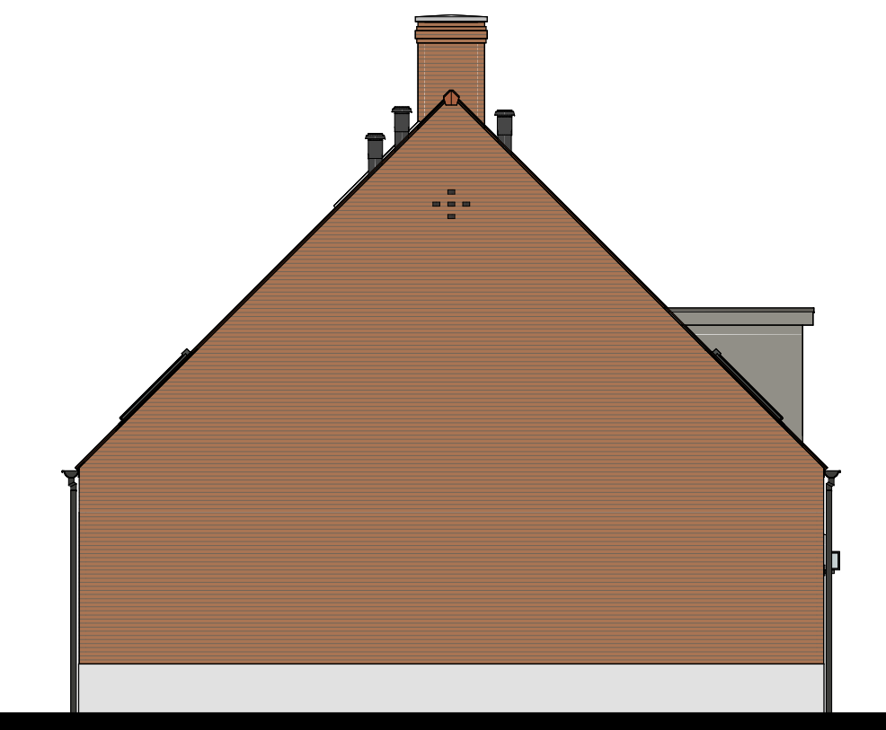
Rechtergevel
