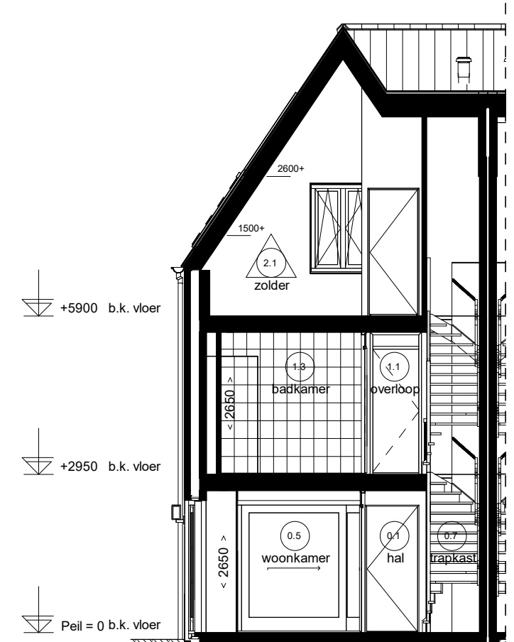
Doorsnede F11.4
