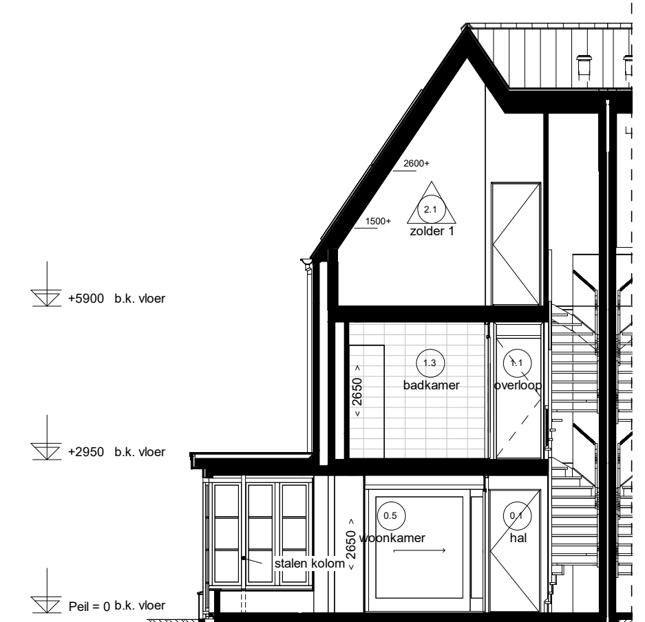
Doorsnede F09.3
