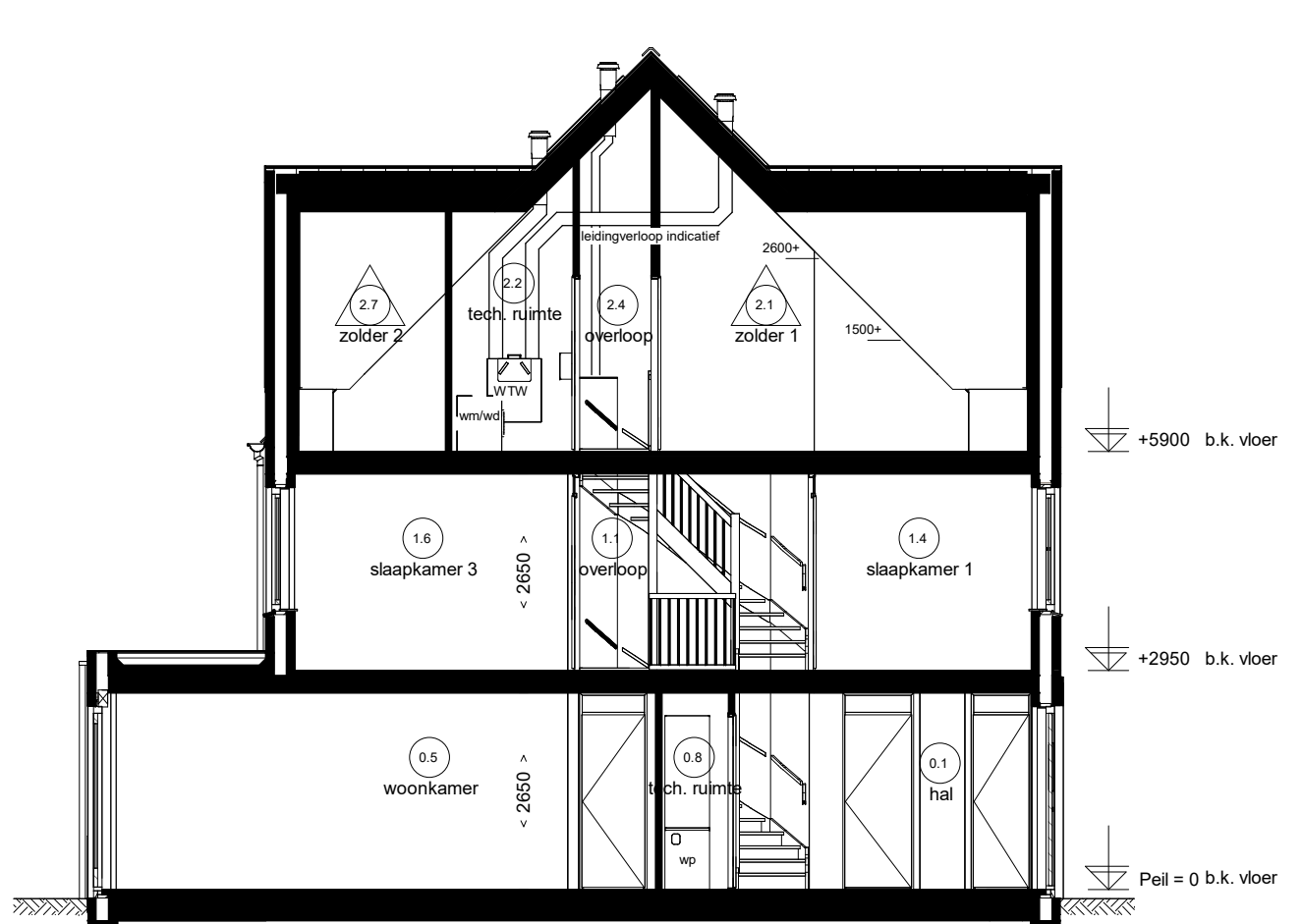
Doorsnede F09.3
