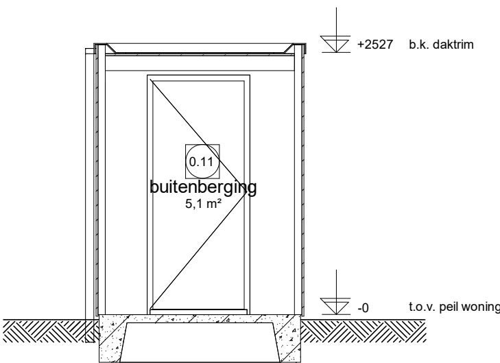
Doorsnede D1.1
