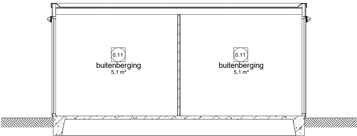
Doorsnede D1.2
