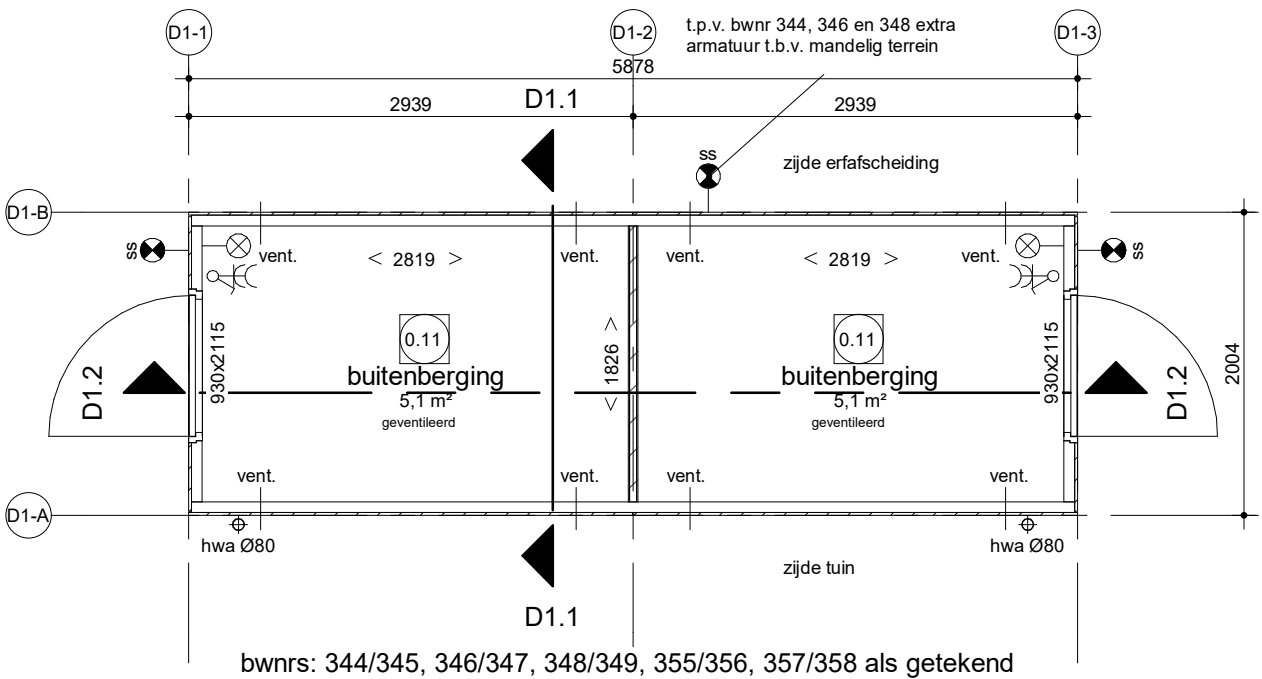
Begane grond
