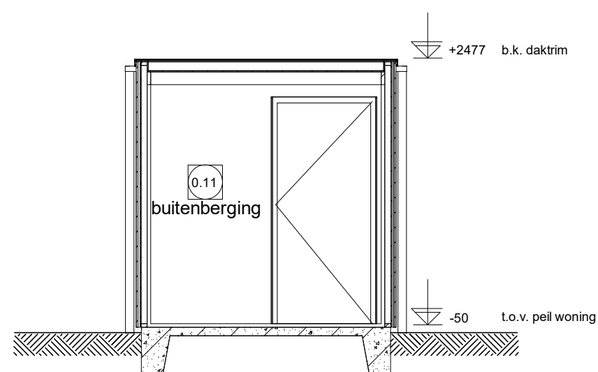
Doorsnede A
