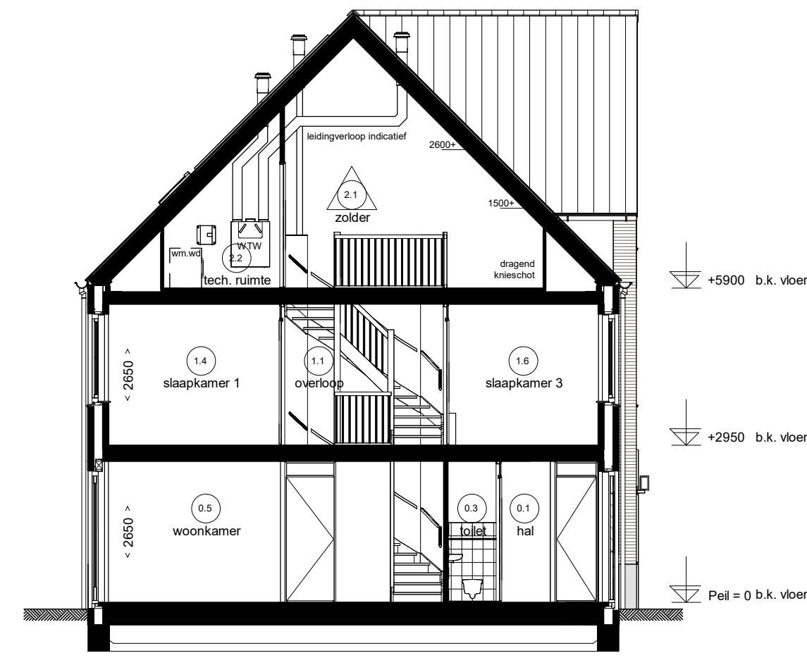
Doorsnede I02.1
