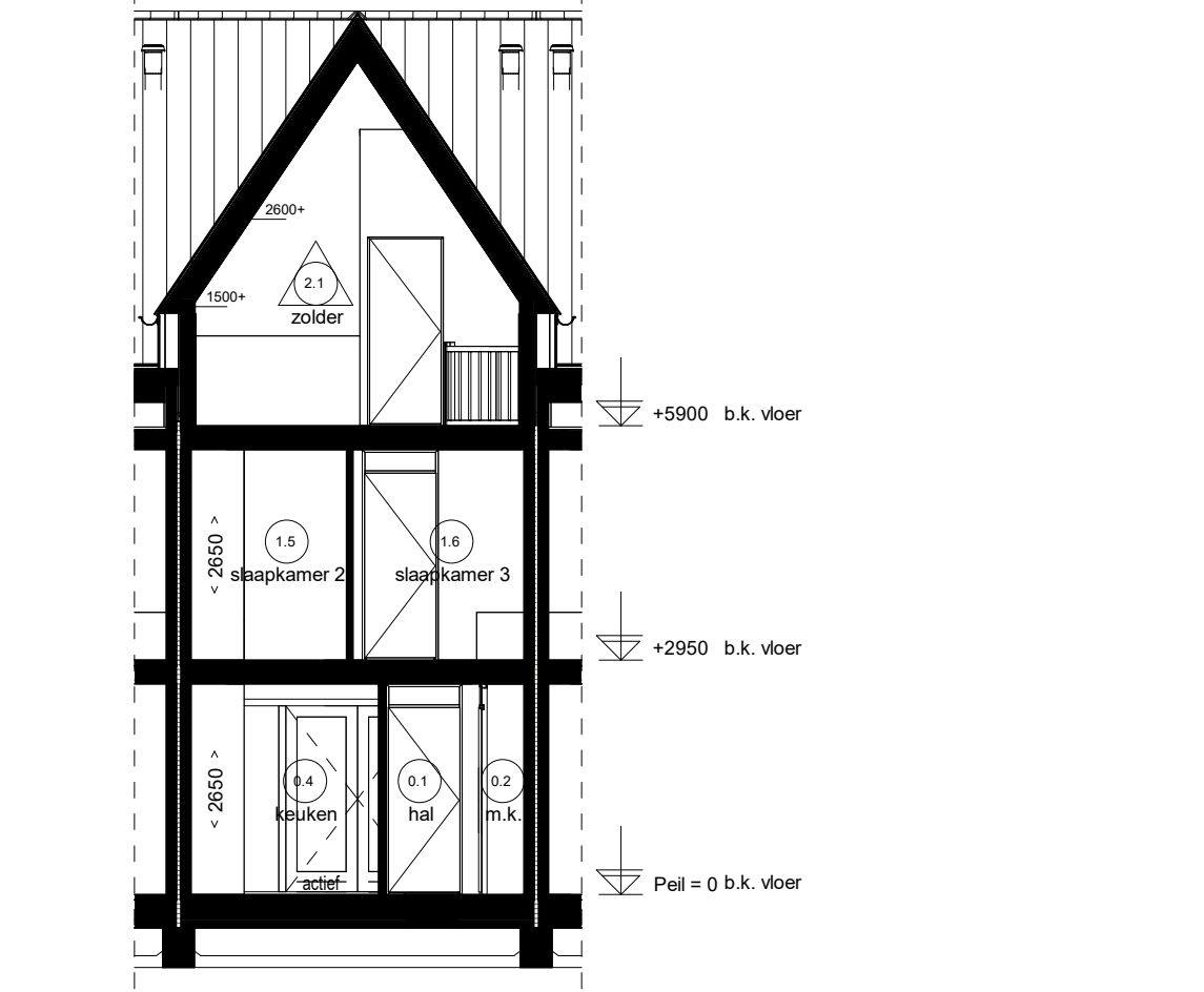
Doorsnede I02.2
